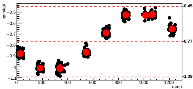
bmod_trim1,cyc=6281
