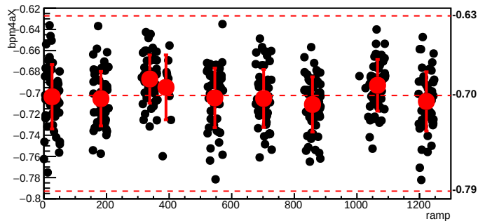
bmod_trim7,cyc=6281
