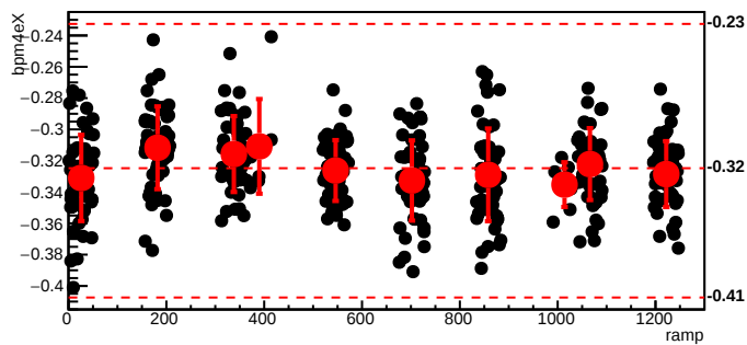
bmod_trim2,cyc=6281
