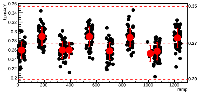
bmod_trim1,cyc=6339
