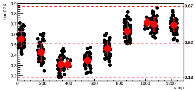
bmod_trim3,cyc=6339
