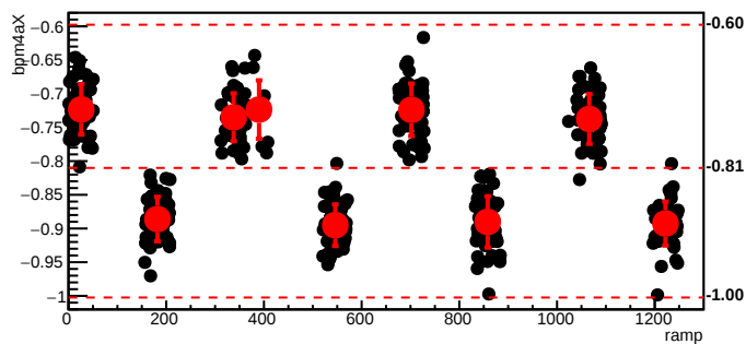
bmod_trim4,cyc=6339
