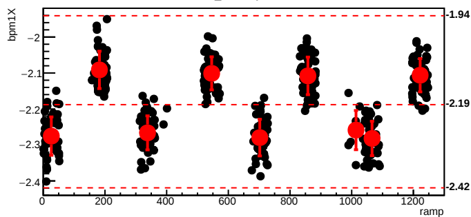
bmod_trim2,cyc=6339
