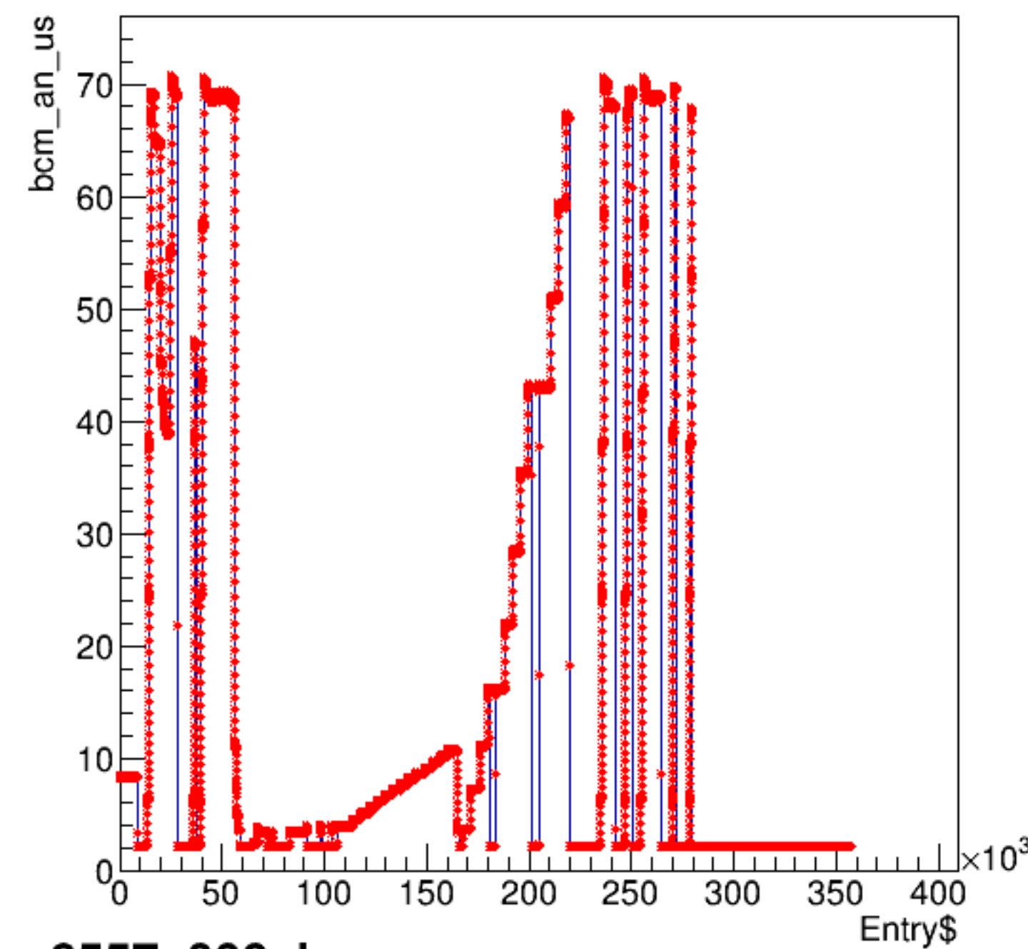
bcm_an_us:Entry$
