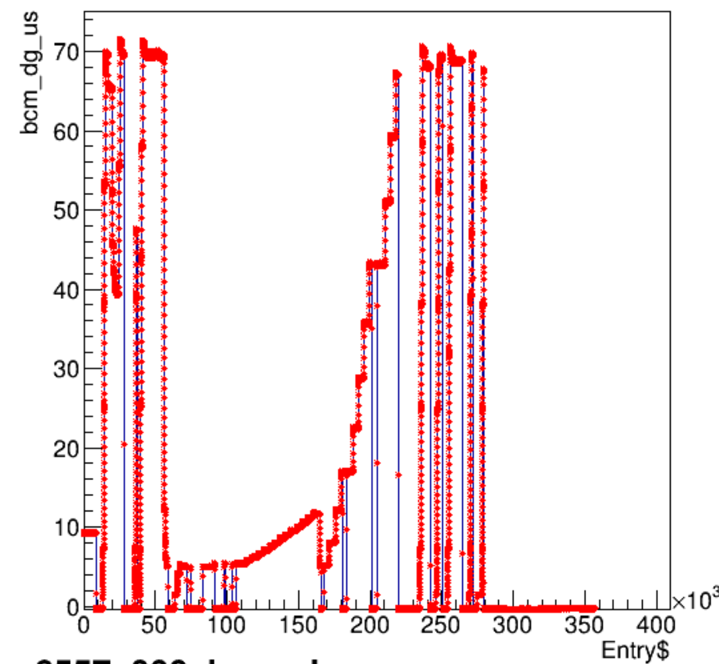
bcm_dg_us:Entry$
