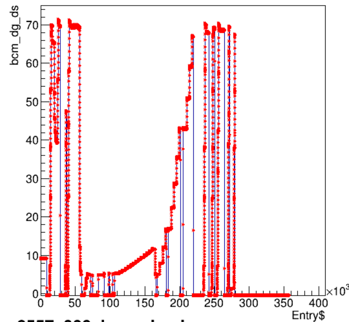
bcm_dg_ds:Entry$
