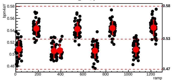
bmod_trim5,cyc=6476
