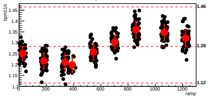
bmod_trim7,cyc=6476
