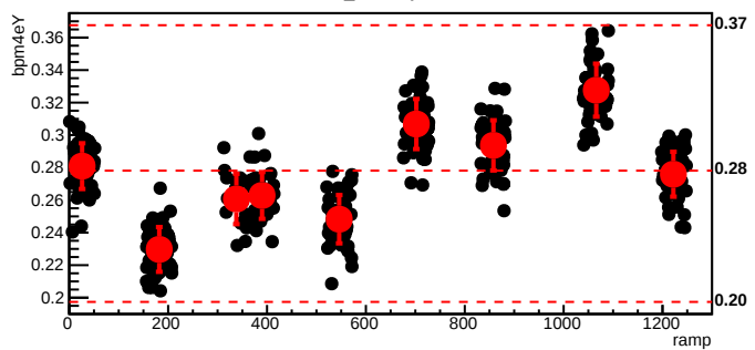
bmod_trim6,cyc=6545
