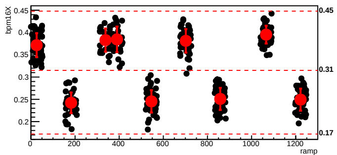
bmod_trim7,cyc=6545
