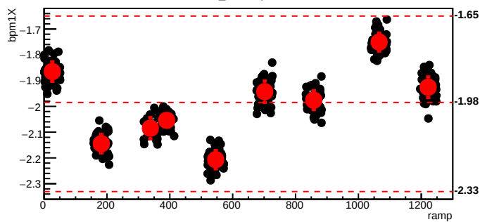
bmod_trim3,cyc=6545
