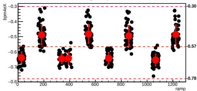
bmod_trim2,cyc=6545
