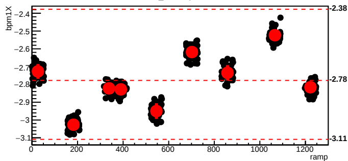
bmod_trim1,cyc=6545
