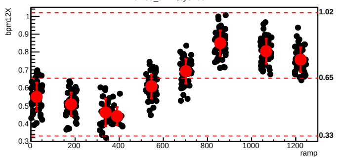
bmod_trim7,cyc=6547
