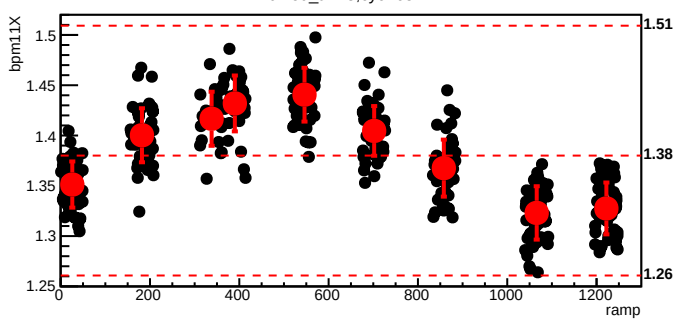
bmod_trim5,cyc=6547
