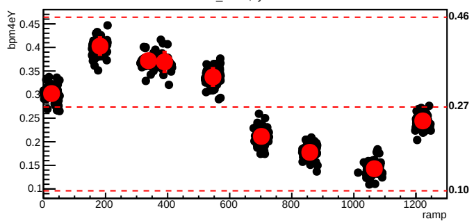
bmod_trim4,cyc=6547
