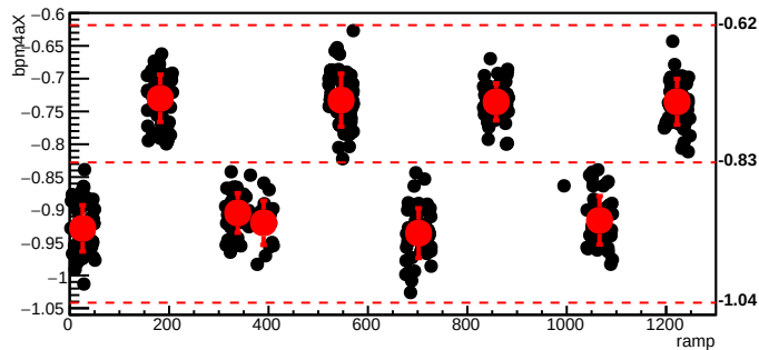
bmod_trim6,cyc=6547
