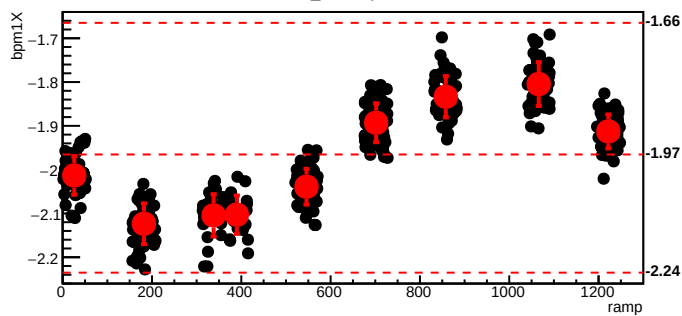
bmod_trim1,cyc=6547
