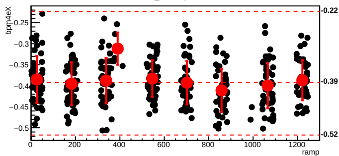
bmod_trim7,cyc=6548
