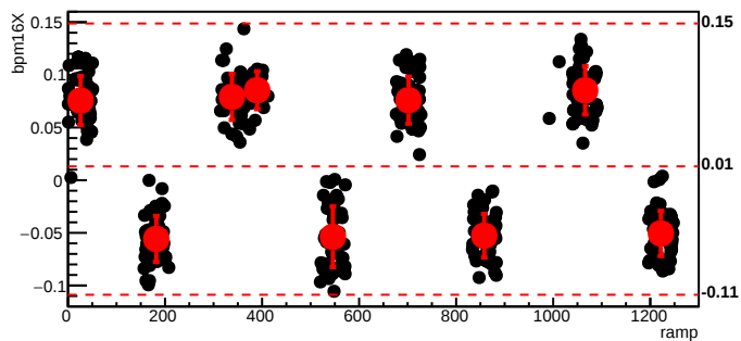
bmod_trim6,cyc=6548
