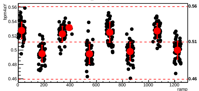
bmod_trim5,cyc=6548
