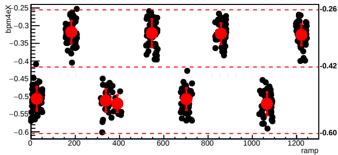
bmod_trim6,cyc=6548
