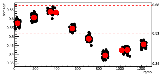
bmod_trim4,cyc=6548
