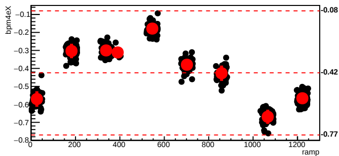
bmod_trim5,cyc=6548
