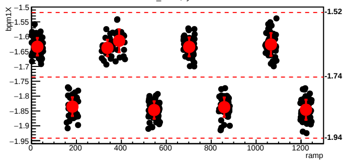
bmod_trim4,cyc=6553
