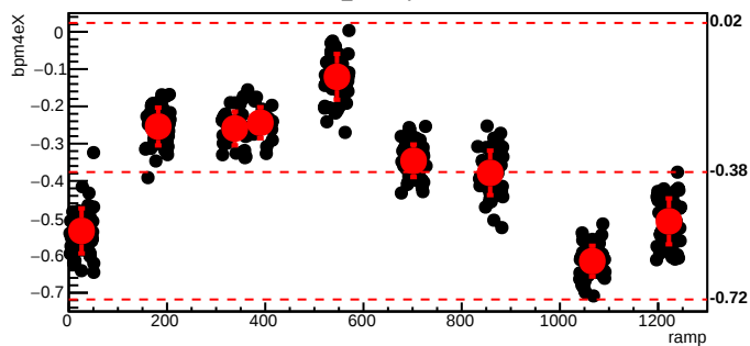
bmod_trim5,cyc=6555
