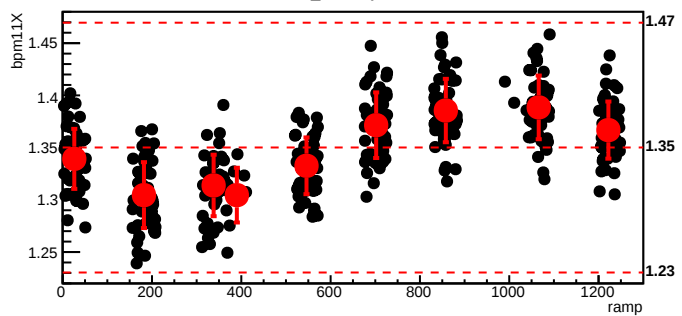
bmod_trim1,cyc=6555
