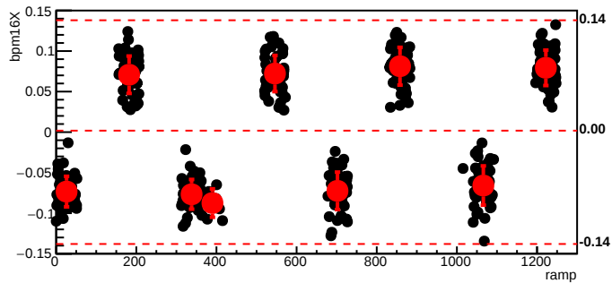
bmod_trim7,cyc=6555
