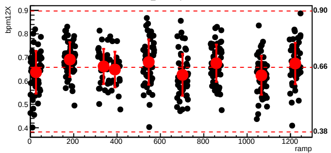
bmod_trim6,cyc=6555
