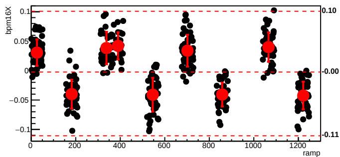
bmod_trim4,cyc=6555
