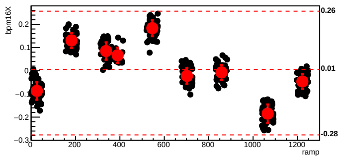
bmod_trim3,cyc=6555
