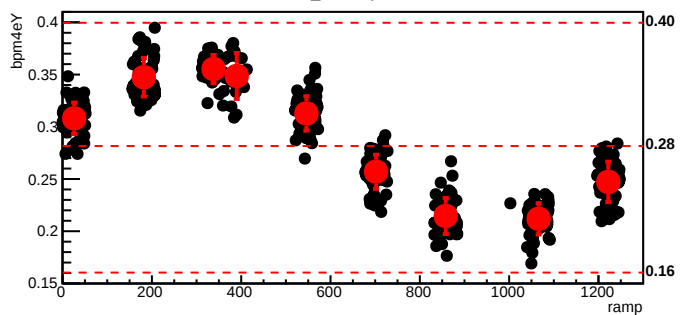
bmod_trim2,cyc=6555
