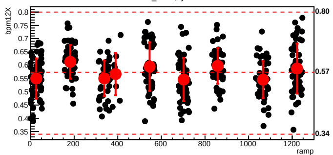
bmod_trim2,cyc=6559
