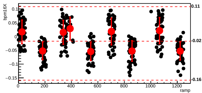
bmod_trim4,cyc=6559
