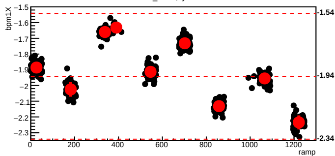
bmod_trim5,cyc=6559
