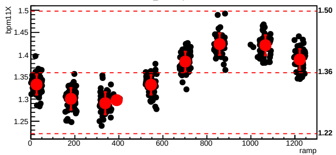
bmod_trim7,cyc=6559
