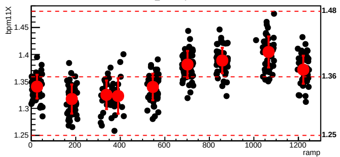
bmod_trim1,cyc=6559
