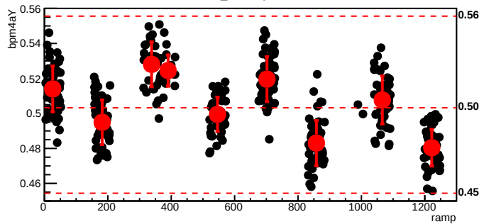
bmod_trim3,cyc=6559
