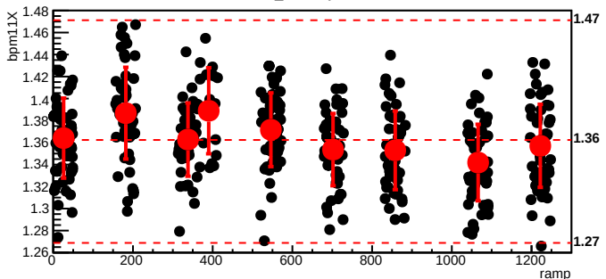
bmod_trim6,cyc=6559
