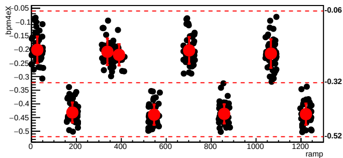
bmod_trim6,cyc=6559
