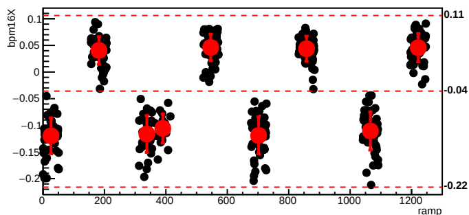
bmod_trim6,cyc=6559
