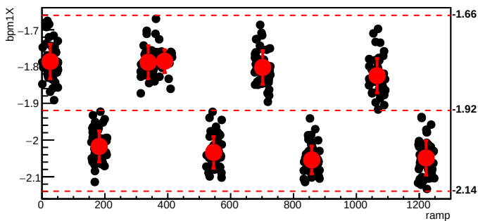
bmod_trim6,cyc=6559
