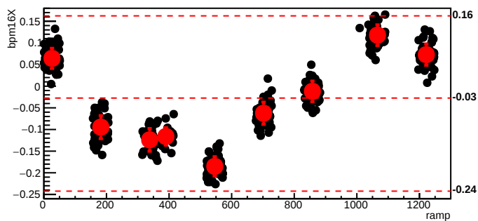
bmod_trim5,cyc=6562
