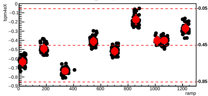
bmod_trim1,cyc=6562
