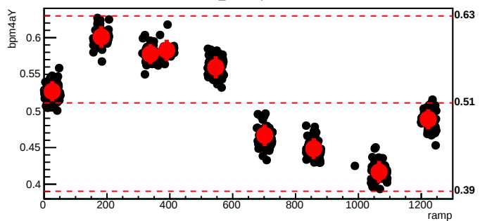
bmod_trim6,cyc=6562
