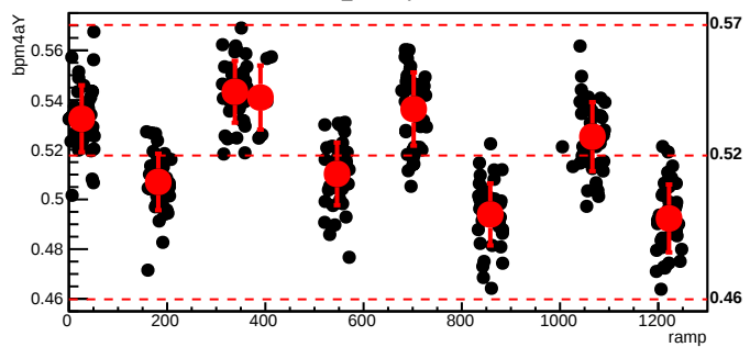
bmod_trim3,cyc=6562
