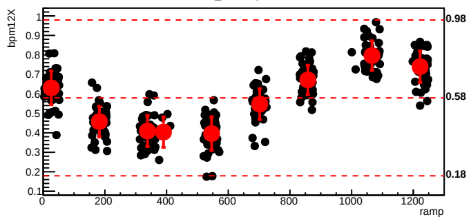
bmod_trim3,cyc=6562
