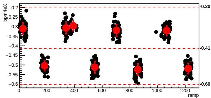
bmod_trim7,cyc=6562
