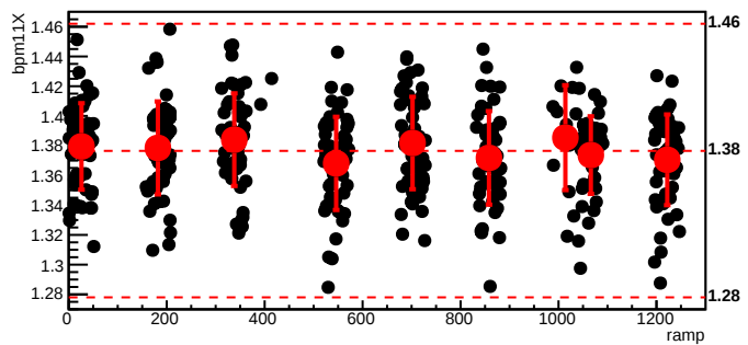
bmod_trim2,cyc=6562
