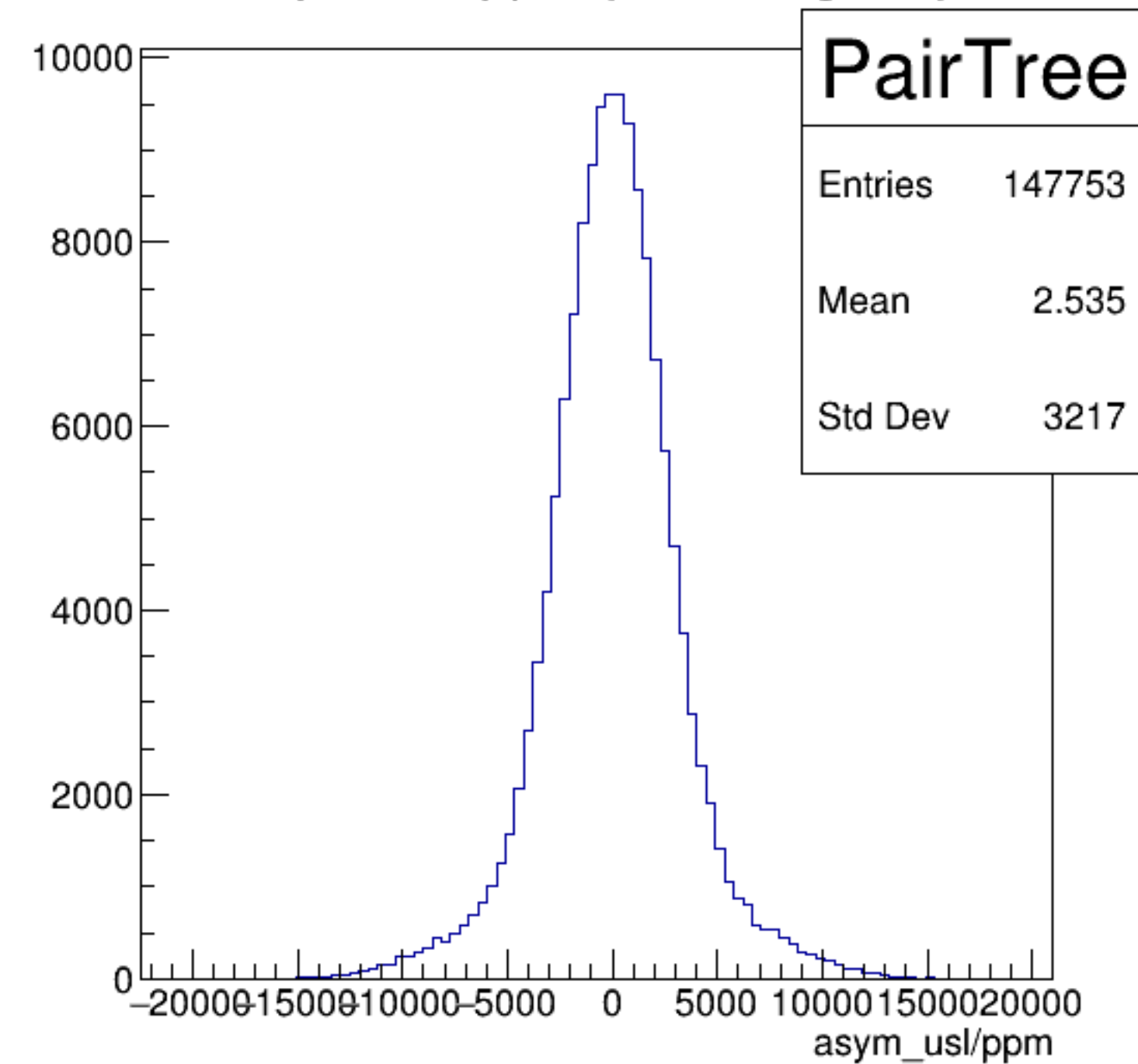
asym_usl/ppm {ErrorFlag==0}
