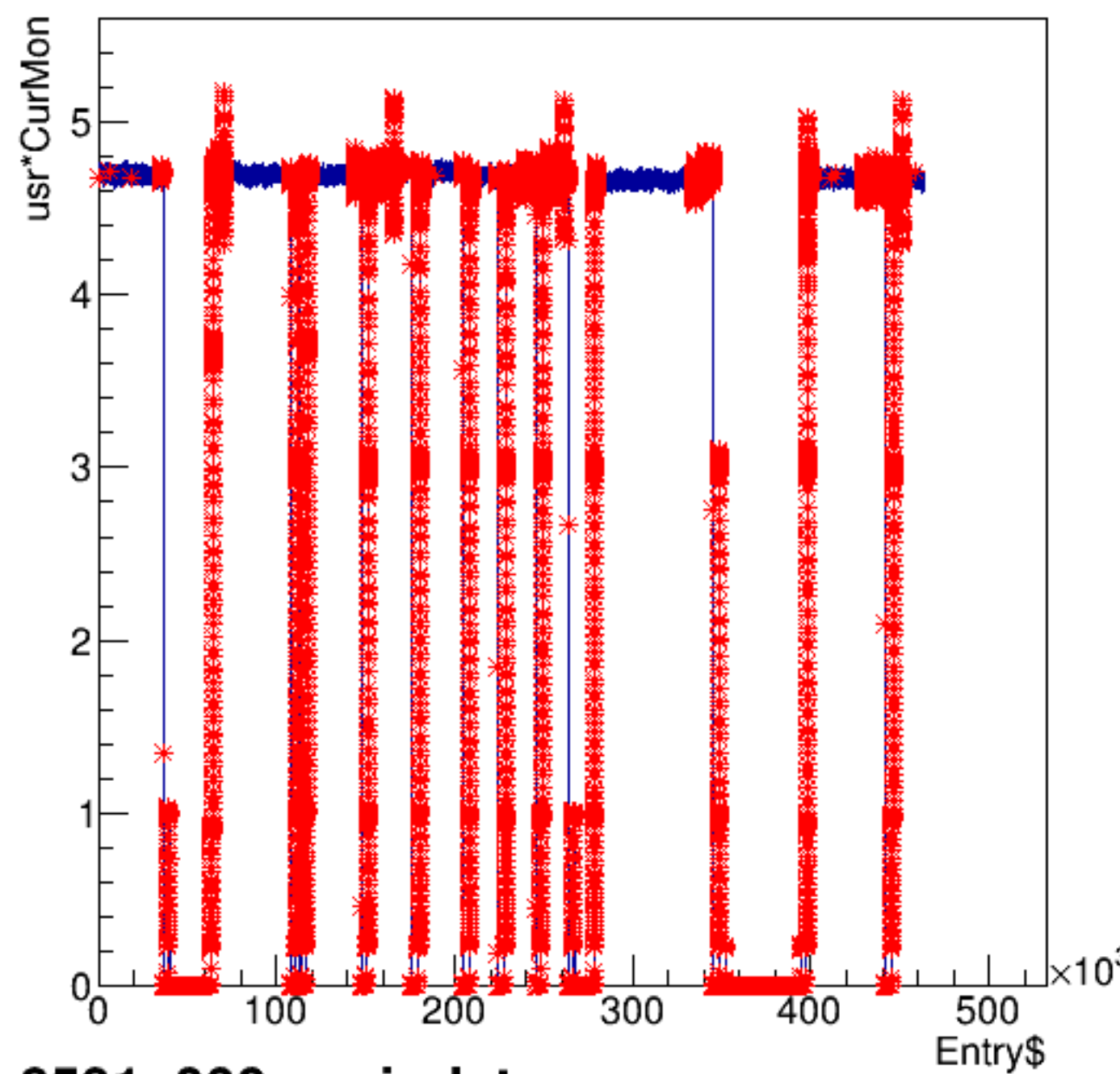
usr*CurMon:Entry$
