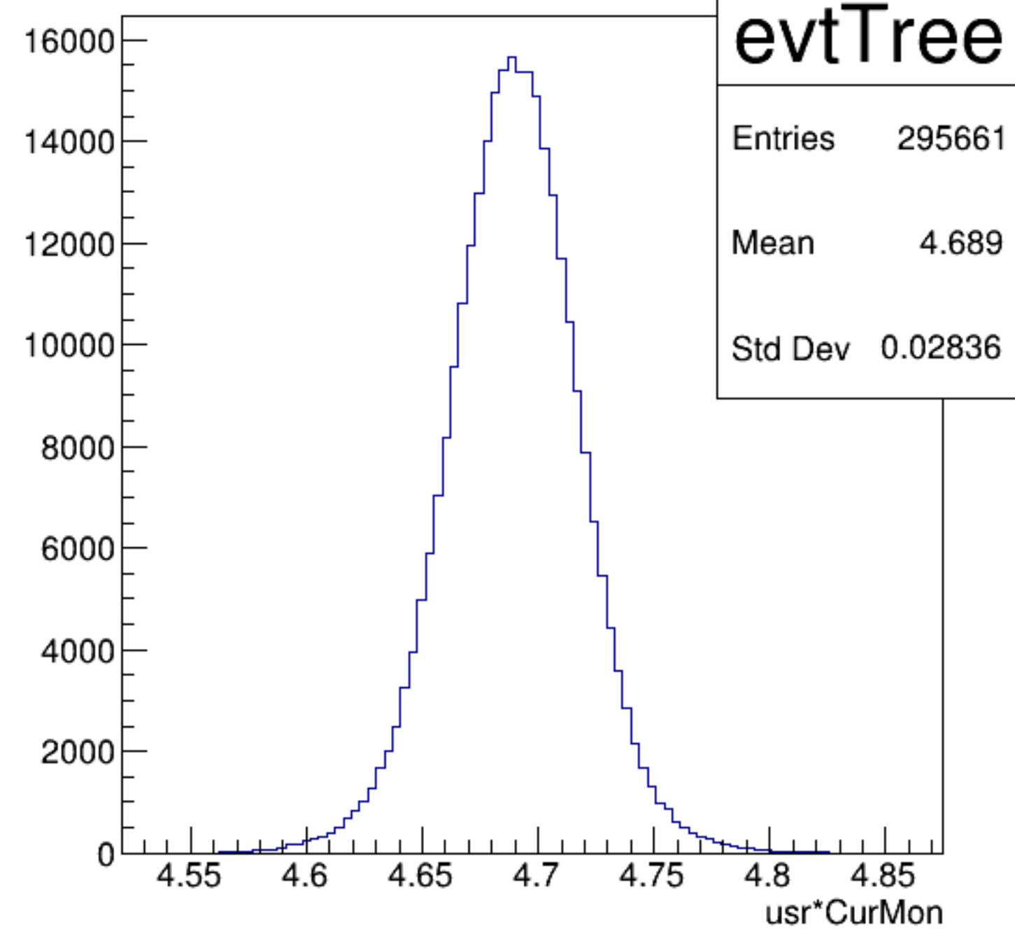
usr*CurMon {ErrorFlag==0}
