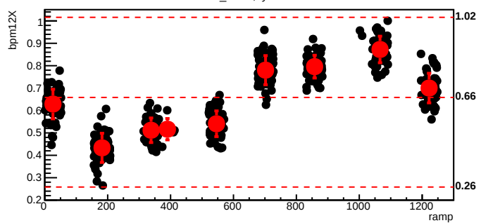
bmod_trim7,cyc=6572
