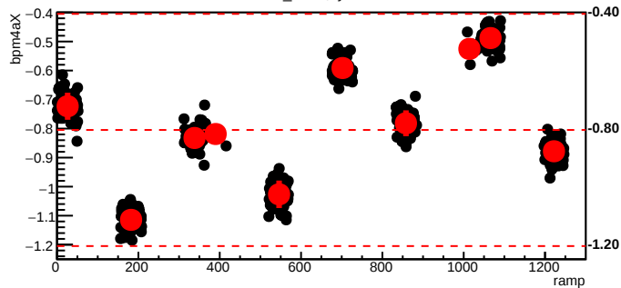
bmod_trim1,cyc=6572
