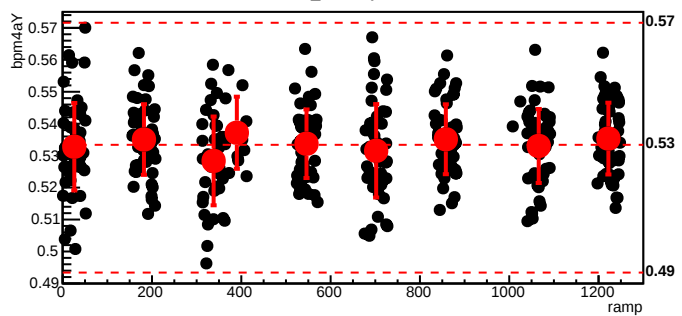
bmod_trim5,cyc=6572
