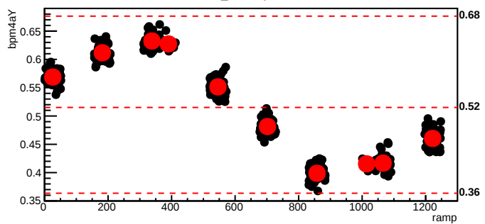
bmod_trim4,cyc=6572
