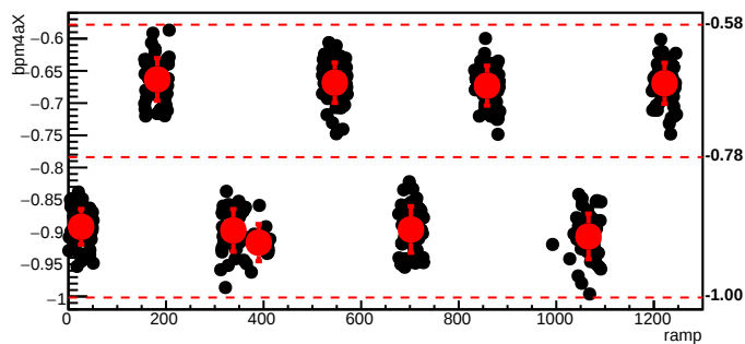
bmod_trim6,cyc=6572
