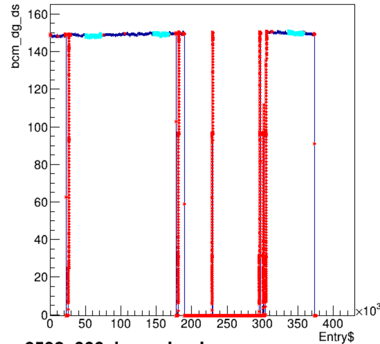
bcm_dg_ds:Entry$
