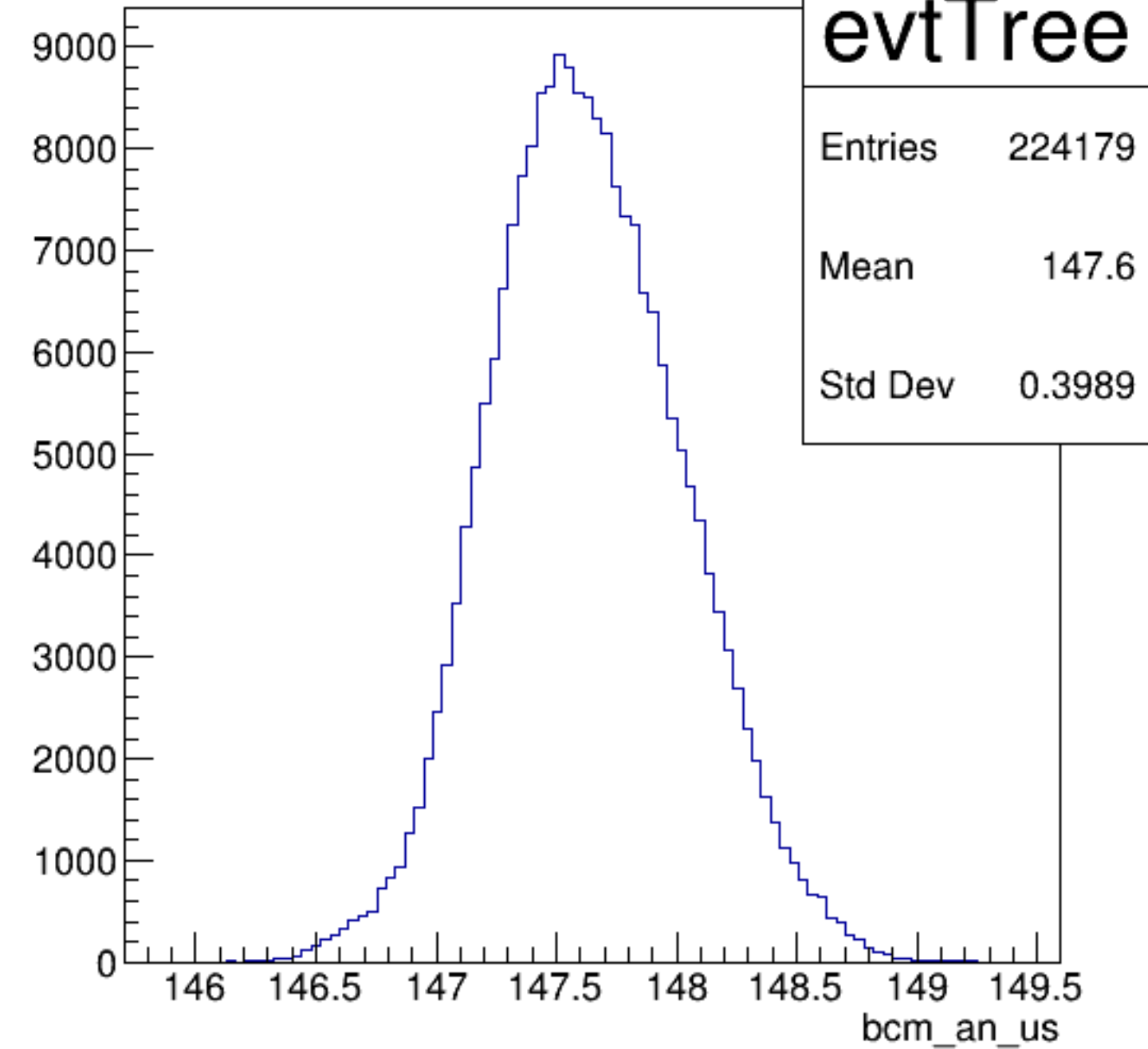
bcm_an_us {ErrorFlag==0}
