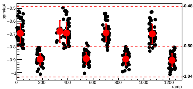
bmod_trim6,cyc=6583
