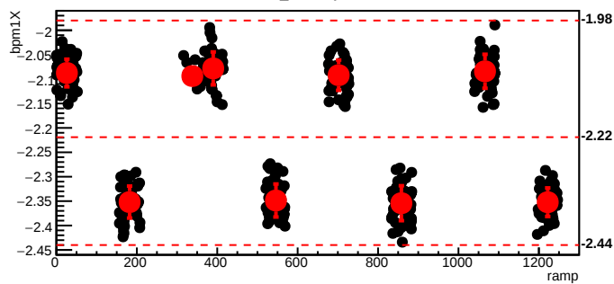
bmod_trim4,cyc=6583
