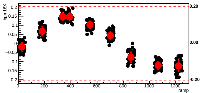
bmod_trim3,cyc=6583
