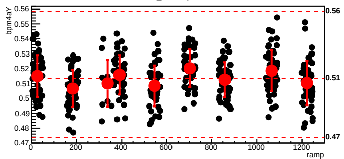
bmod_trim7,cyc=6583
