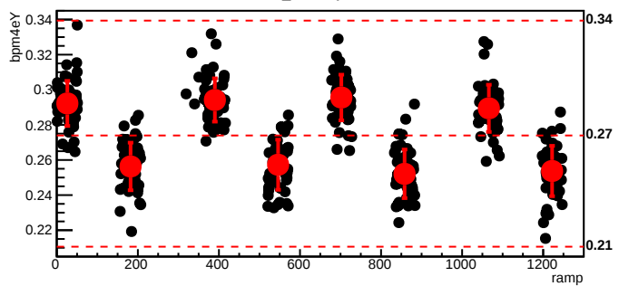
bmod_trim1,cyc=6583
