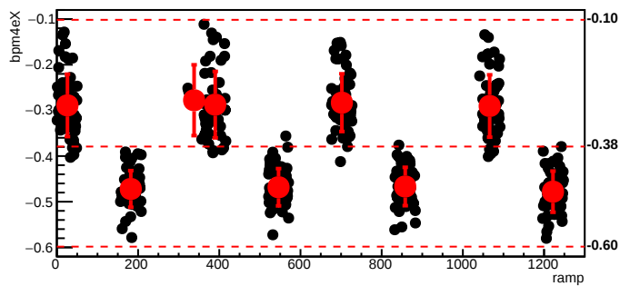
bmod_trim6,cyc=6583
