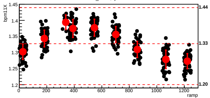
bmod_trim5,cyc=6583
