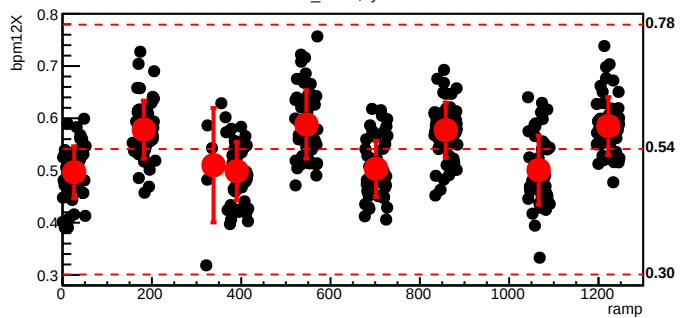
bmod_trim2,cyc=6583
