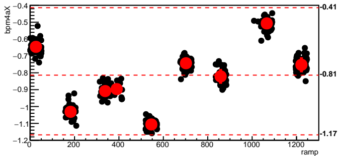
bmod_trim3,cyc=6580
