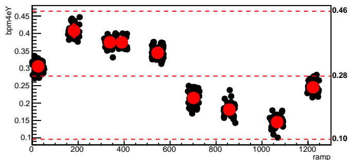
bmod_trim4,cyc=6580
