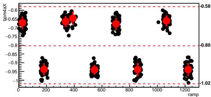
bmod_trim6,cyc=6580
