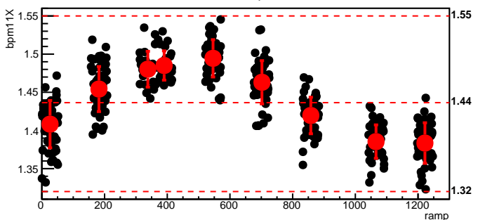
bmod_trim5,cyc=6580
