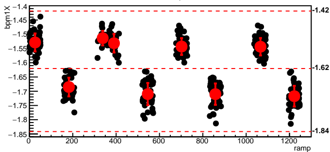
bmod_trim7,cyc=6580
