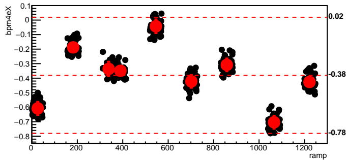
bmod_trim5,cyc=6580
