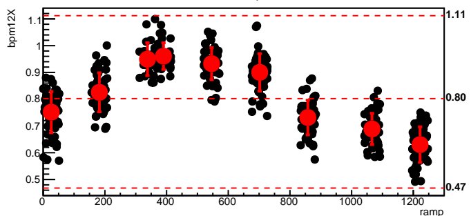
bmod_trim5,cyc=6580
