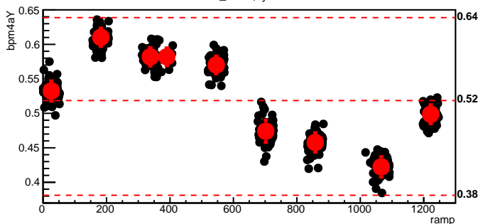
bmod_trim2,cyc=6580
