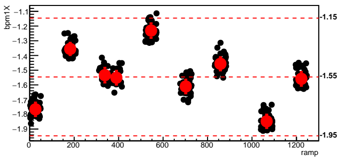
bmod_trim5,cyc=6580
