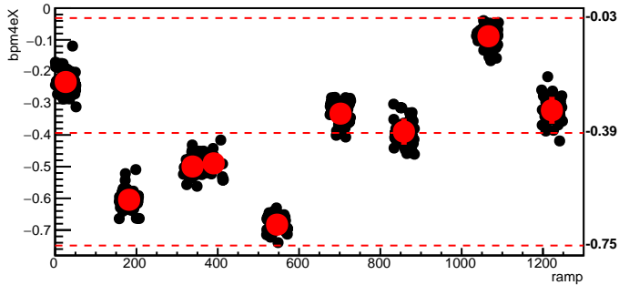
bmod_trim3,cyc=6580
