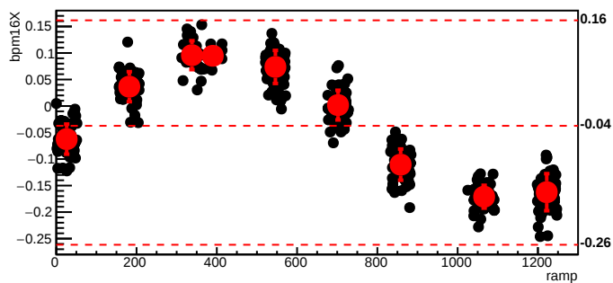
bmod_trim3,cyc=6593
