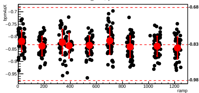
bmod_trim2,cyc=6593
