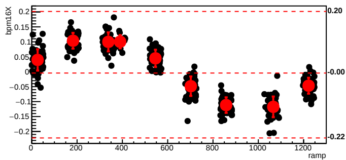
bmod_trim1,cyc=6593
