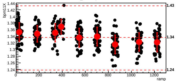
bmod_trim6,cyc=6593
