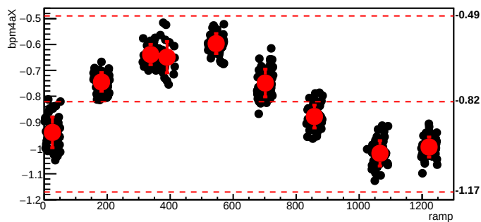
bmod_trim5,cyc=6593
