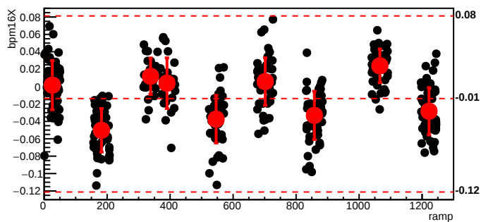
bmod_trim7,cyc=6593
