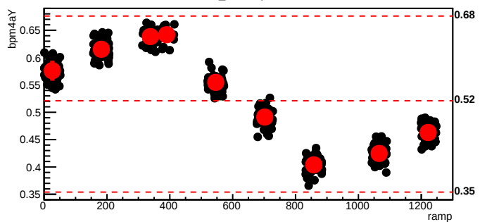
bmod_trim4,cyc=6593
