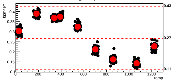
bmod_trim4,cyc=6603
