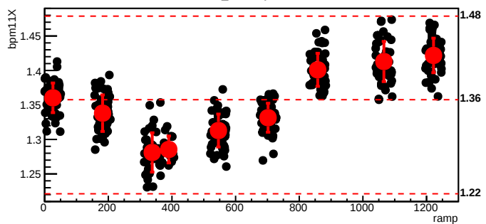
bmod_trim3,cyc=6603
