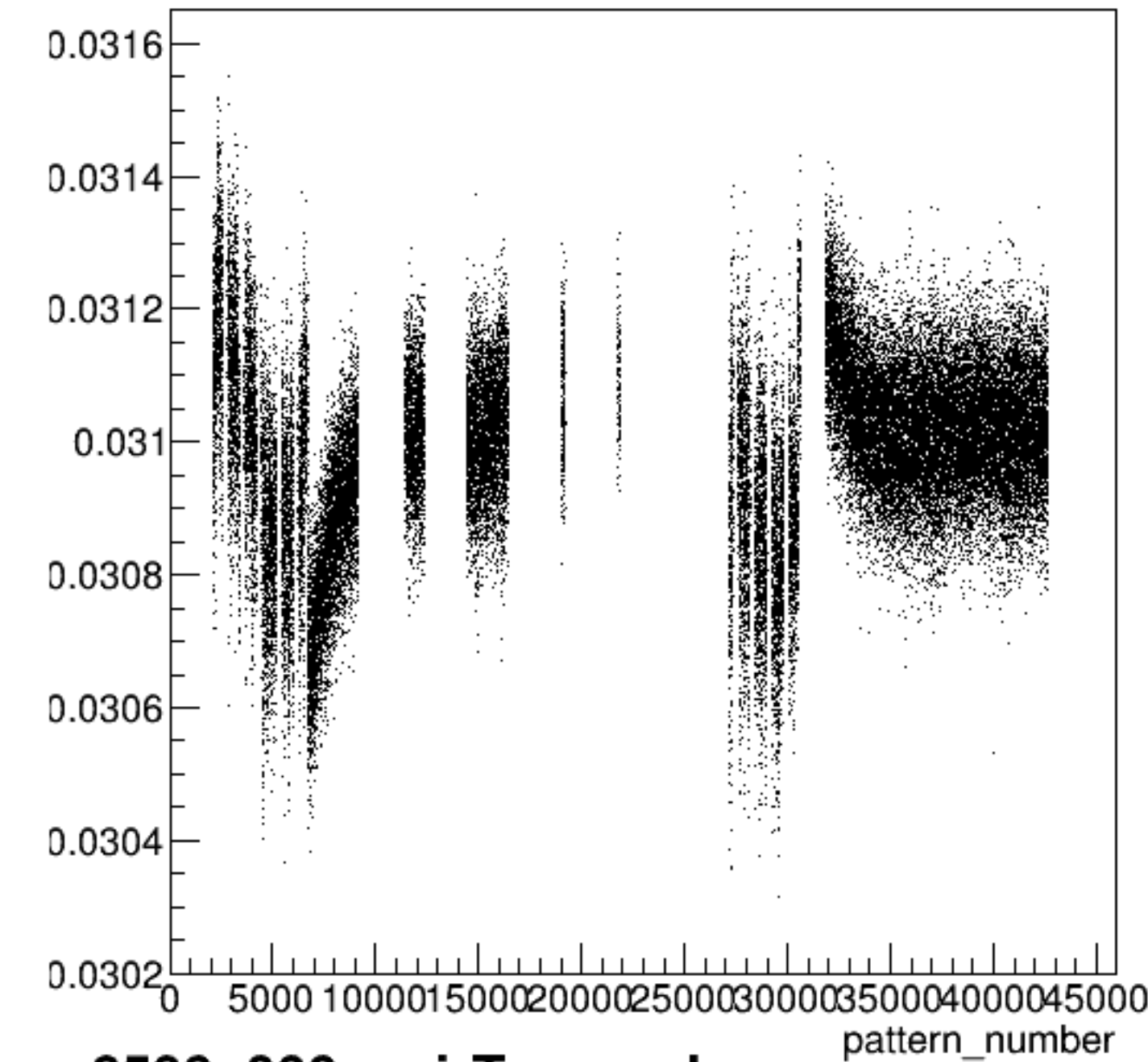
yield_usl:pattern_number {ErrorFlag==0}
