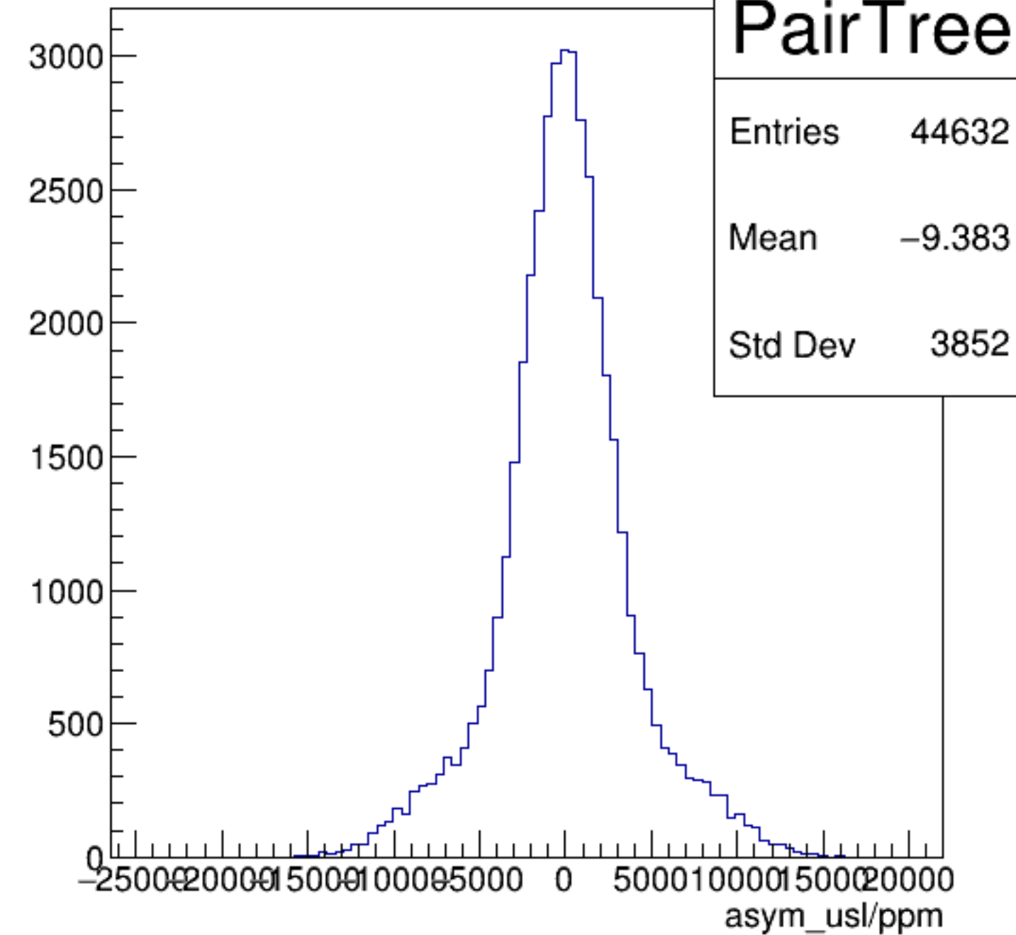
asym_usl/ppm {ErrorFlag==0}
