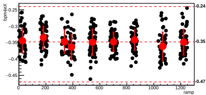
bmod_trim6,cyc=6605
