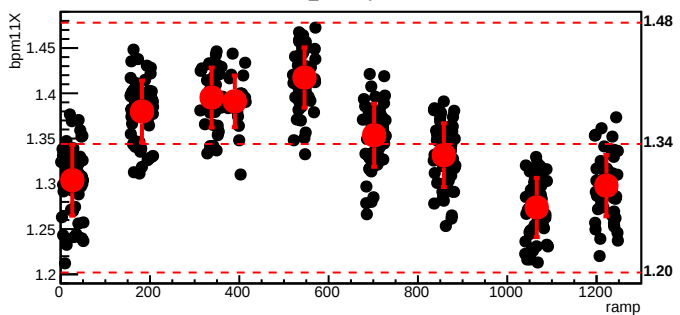
bmod_trim5,cyc=6605
