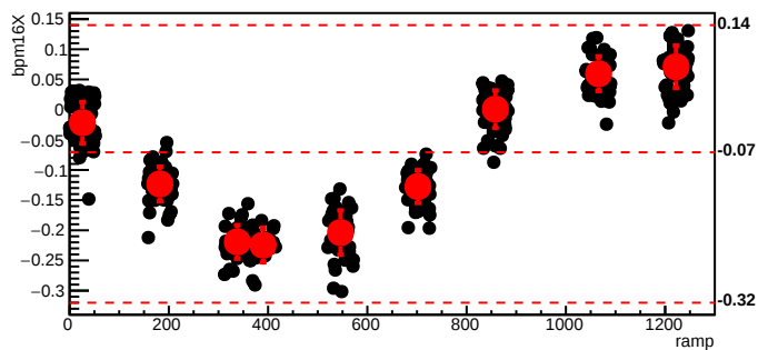
bmod_trim5,cyc=6605
