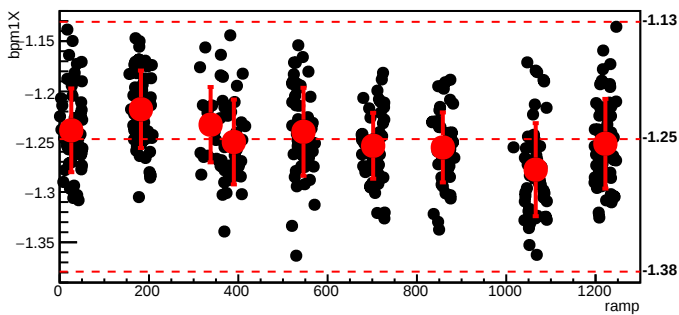
bmod_trim6,cyc=6605
