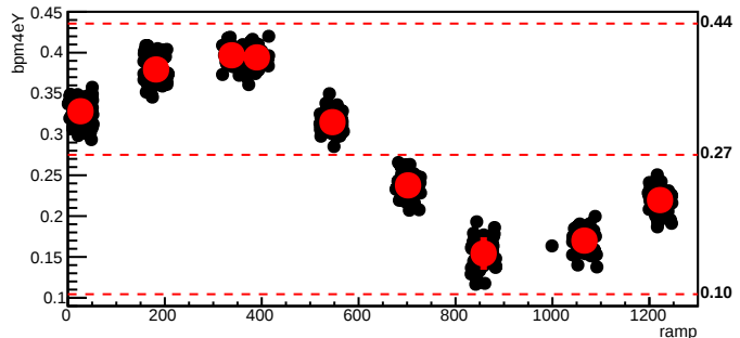
bmod_trim4,cyc=6605
