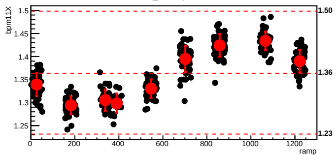
bmod_trim7,cyc=6605
