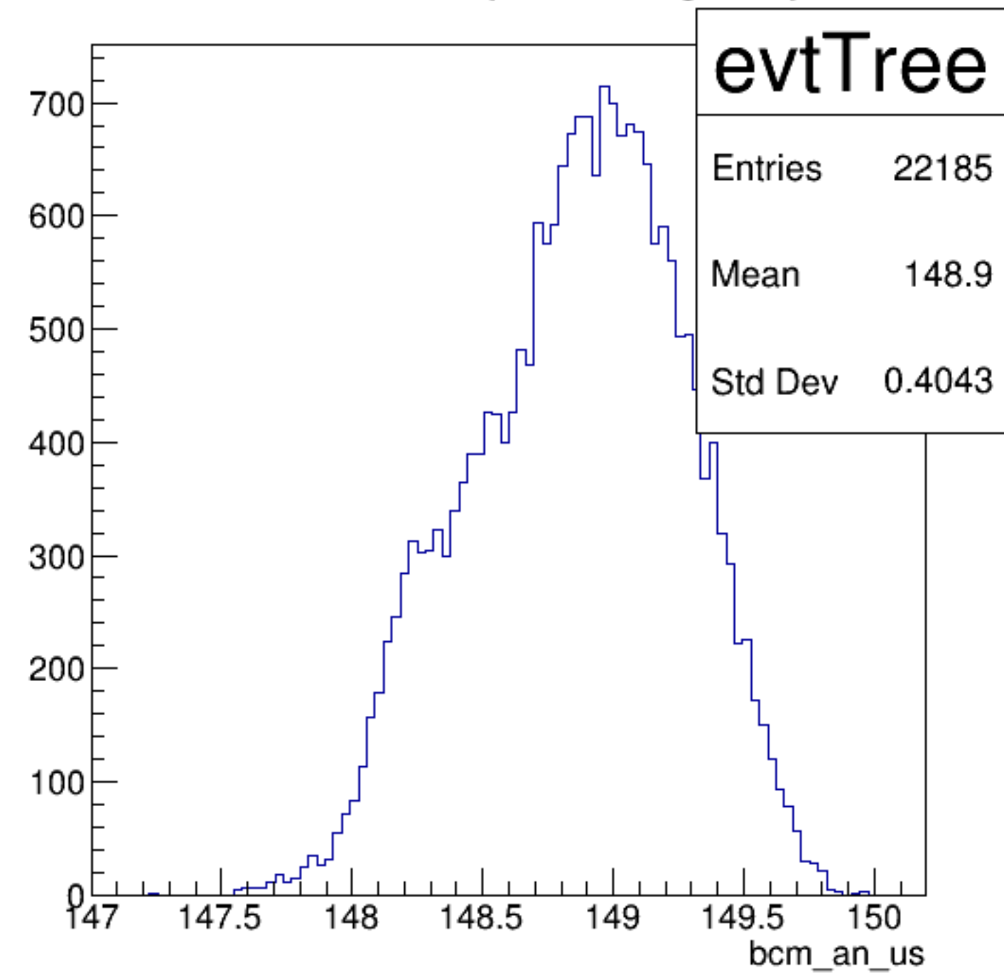
bcm_an_us {ErrorFlag==0}
