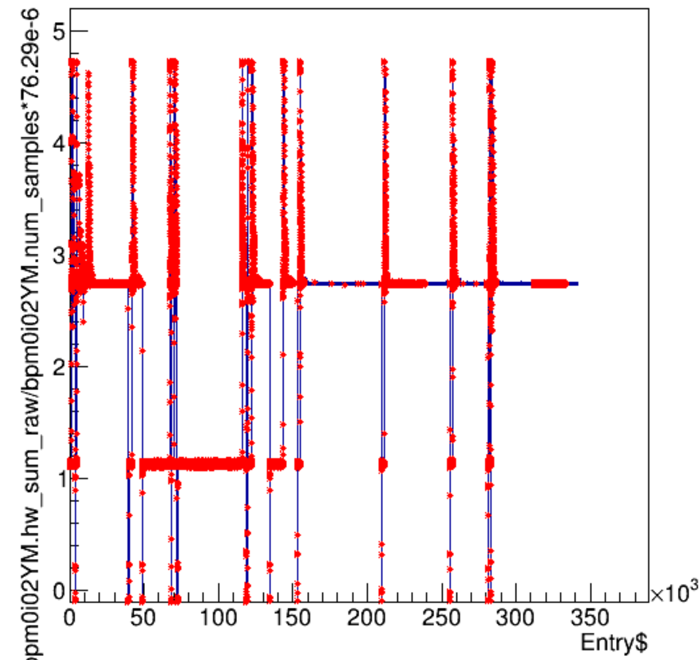
bpm0i02YM.hw_sum_raw/bpm0i02YM.num_samples*76.29e-6:Entry$
