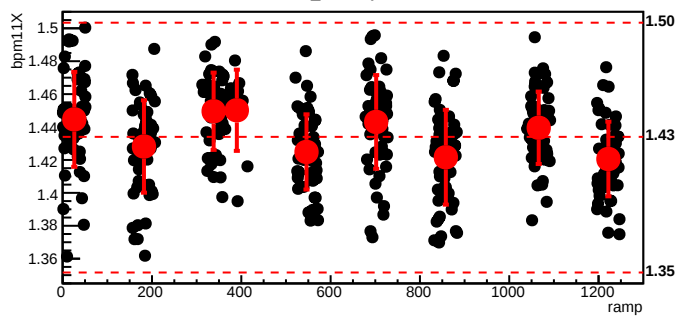
bmod_trim2,cyc=6687
