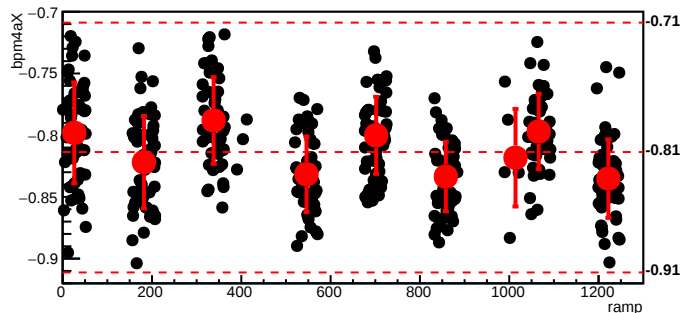
bmod_trim6,cyc=6687
