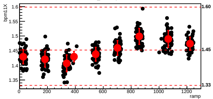
bmod_trim1,cyc=6687
