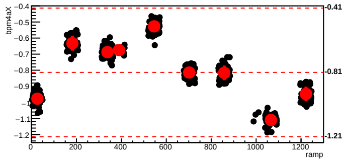
bmod_trim5,cyc=6687
