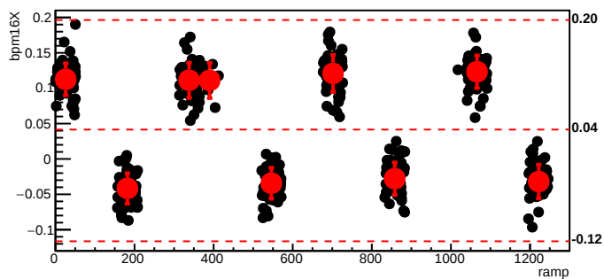
bmod_trim7,cyc=6687
