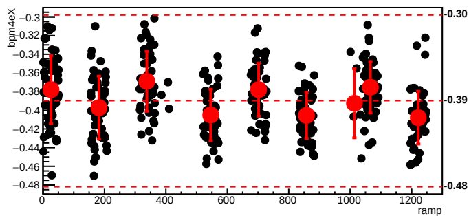
bmod_trim6,cyc=6687
