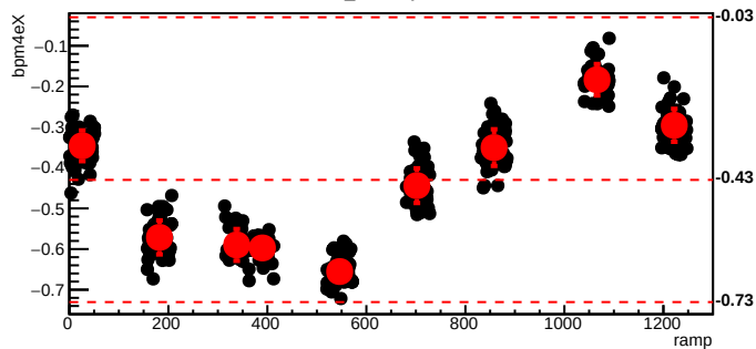
bmod_trim3,cyc=6694
