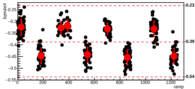
bmod_trim6,cyc=6694
