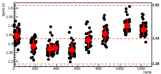
bmod_trim3,cyc=6694
