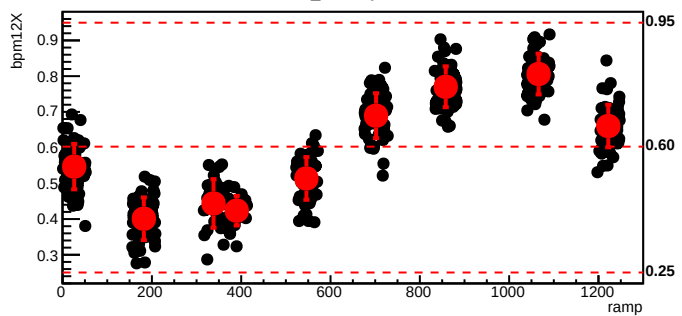
bmod_trim7,cyc=6694
