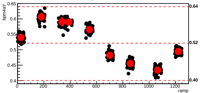
bmod_trim6,cyc=6694
