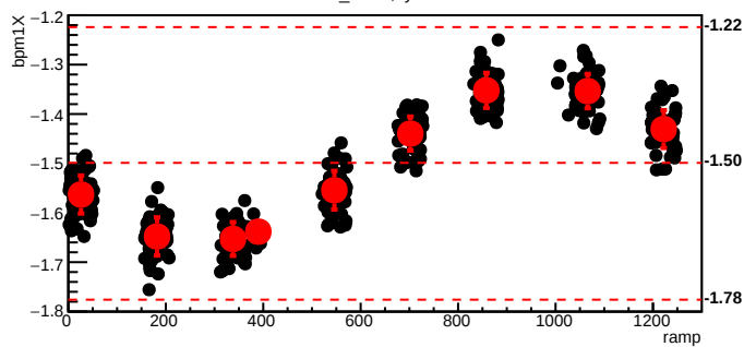
bmod_trim1,cyc=6698
