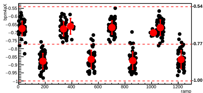
bmod_trim5,cyc=6698
