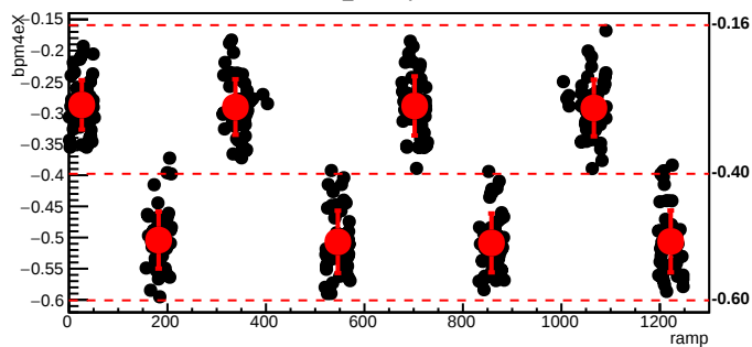
bmod_trim4,cyc=6698
