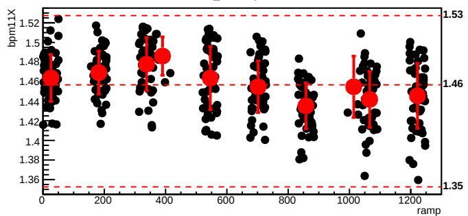
bmod_trim6,cyc=6698
