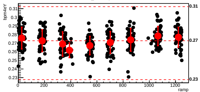
bmod_trim5,cyc=6697
