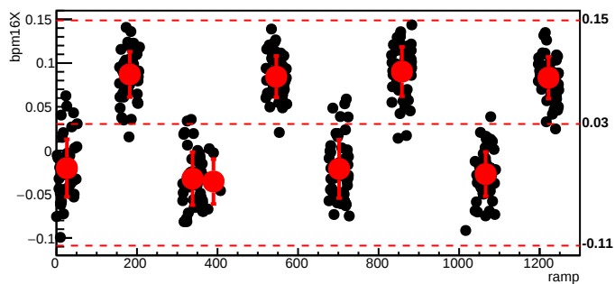
bmod_trim6,cyc=6697
