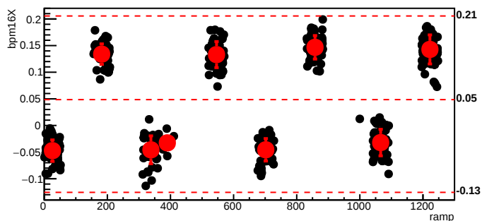
bmod_trim7,cyc=6697
