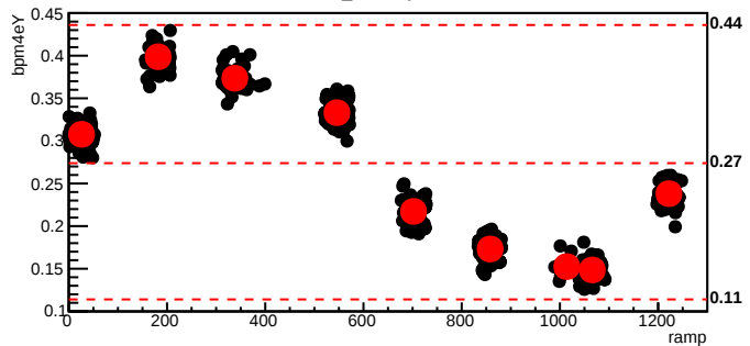
bmod_trim4,cyc=6697
