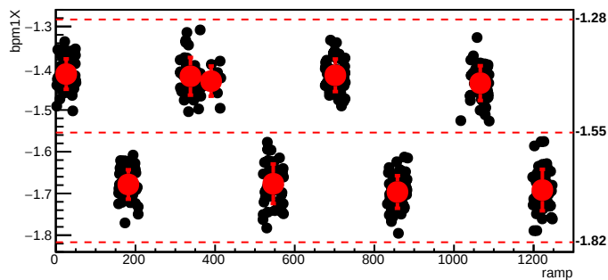
bmod_trim7,cyc=6697
