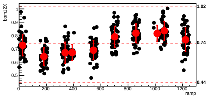
bmod_trim1,cyc=6697
