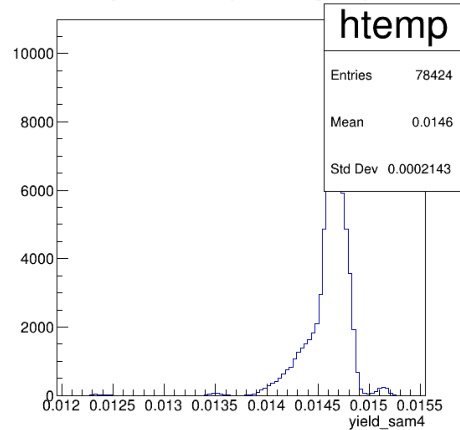
yield_sam4 {ErrorFlag==0}
