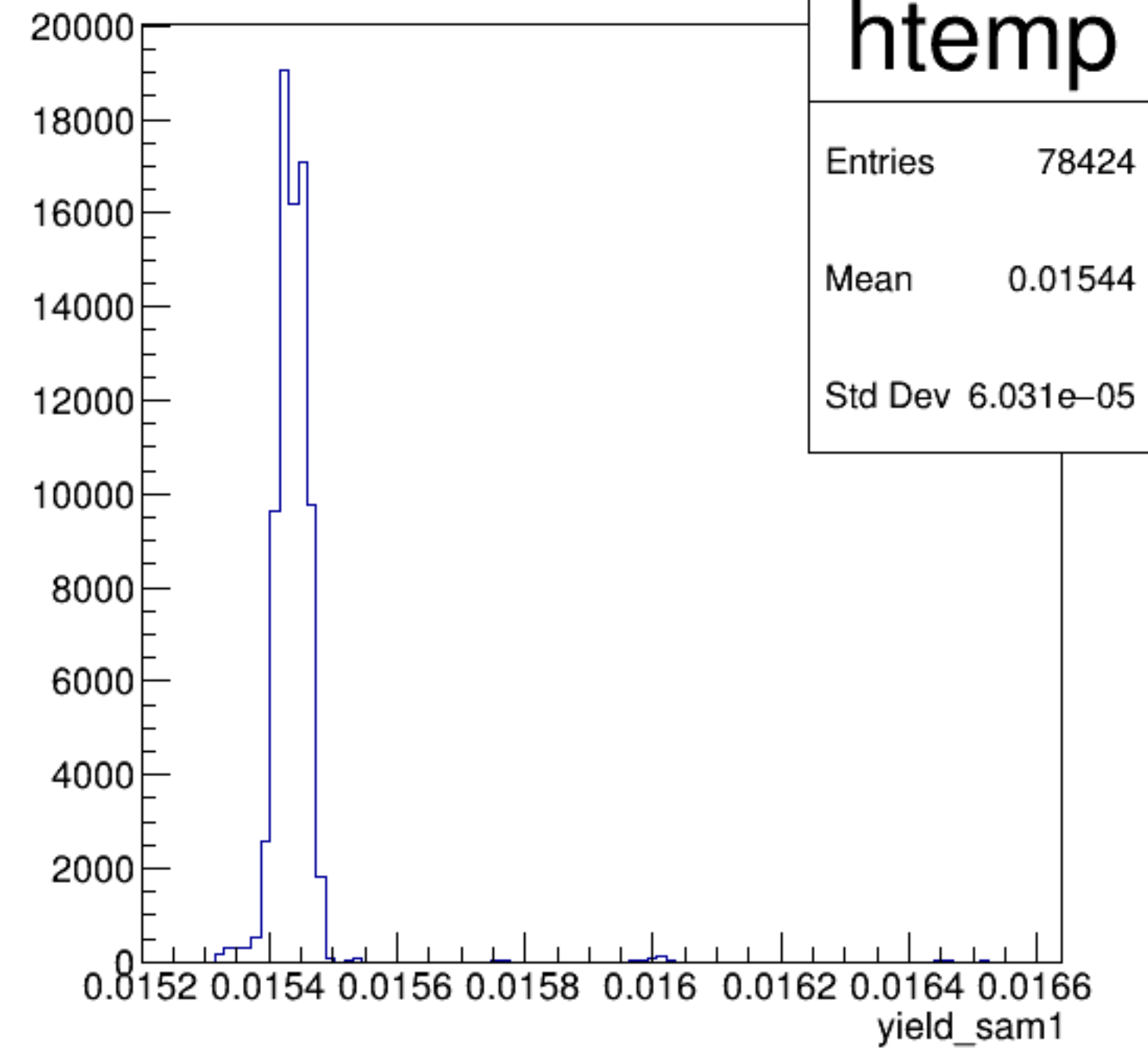
yield_sam1 {ErrorFlag==0}
