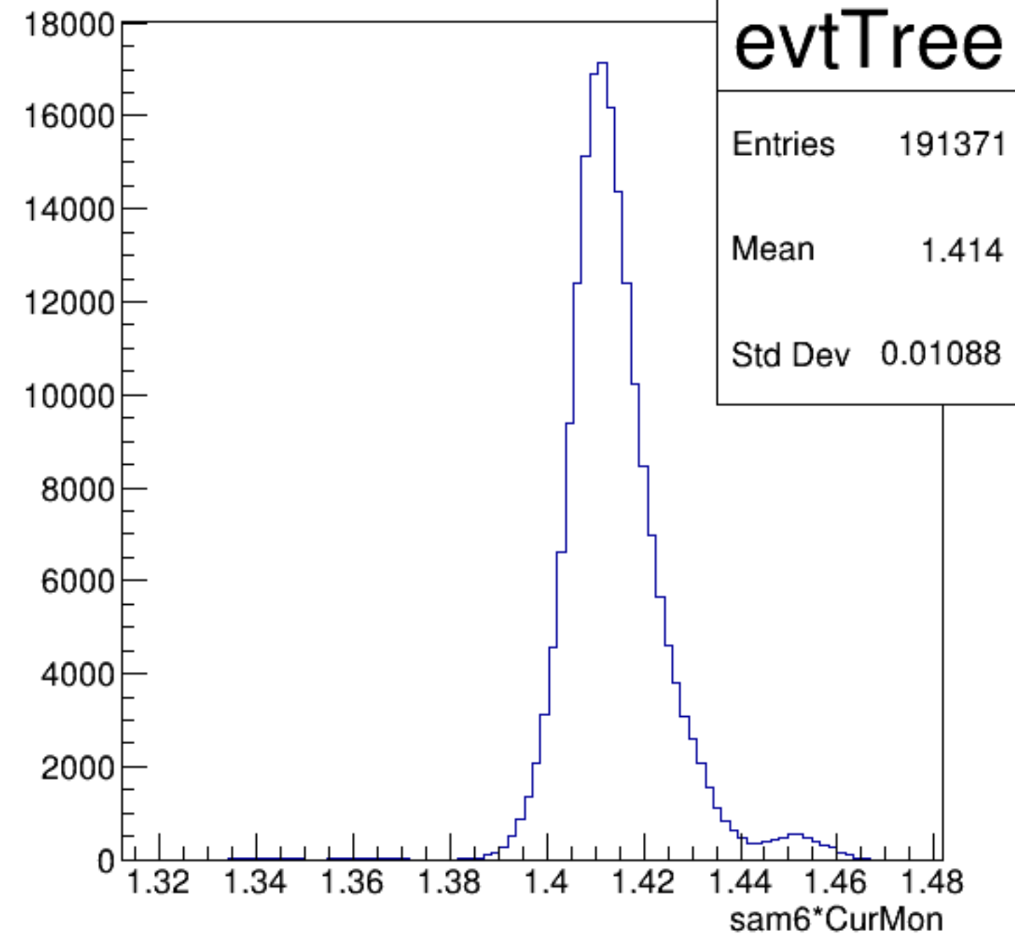
sam6*CurMon {ErrorFlag==0}
