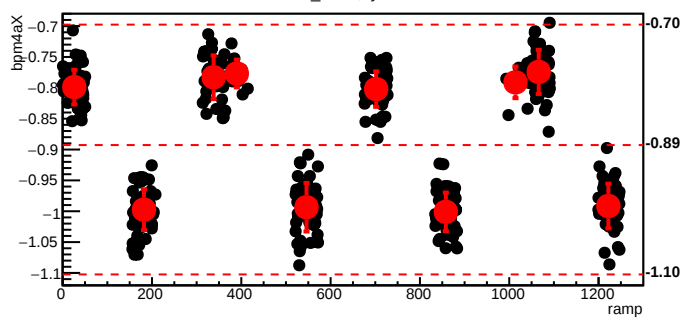
bmod_trim2,cyc=6712
