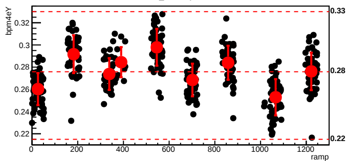
bmod_trim3,cyc=6712
