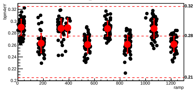
bmod_trim1,cyc=6712
