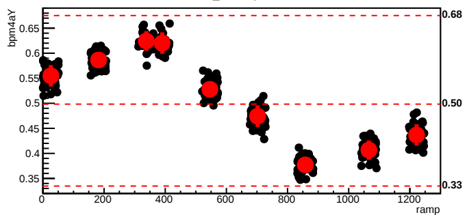
bmod_trim4,cyc=6712
