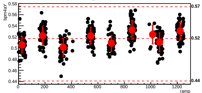
bmod_trim7,cyc=6712
