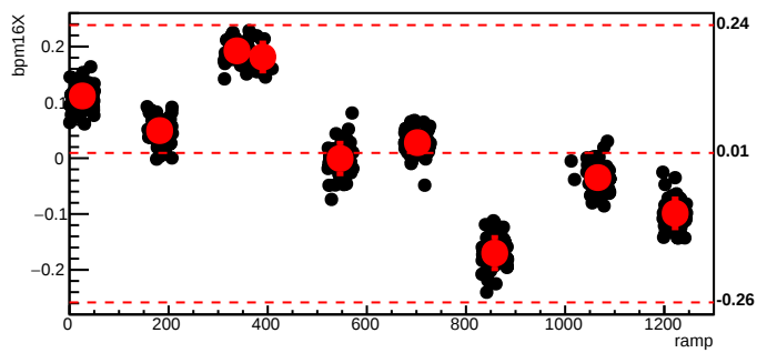
bmod_trim1,cyc=6712
