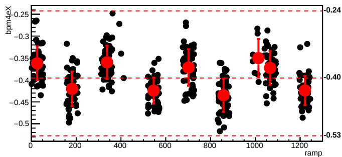
bmod_trim7,cyc=6712
