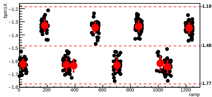
bmod_trim2,cyc=6715
