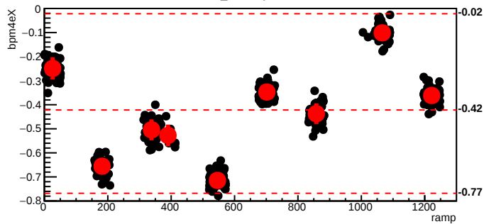
bmod_trim3,cyc=6715
