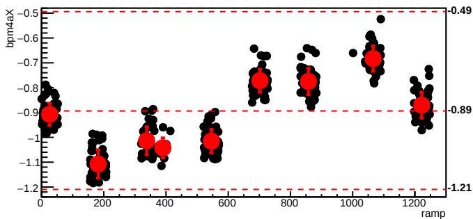
bmod_trim1,cyc=6715
