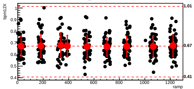
bmod_trim4,cyc=6715
