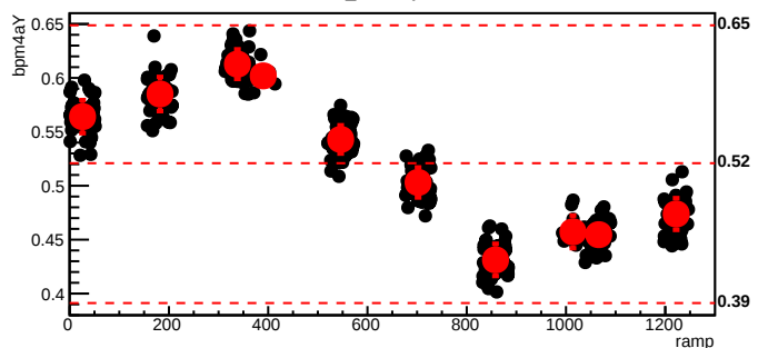
bmod_trim2,cyc=6715
