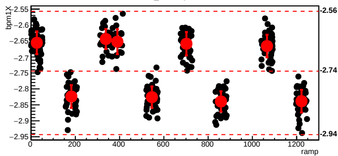
bmod_trim2,cyc=6764
