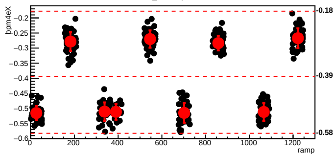
bmod_trim4,cyc=6764
