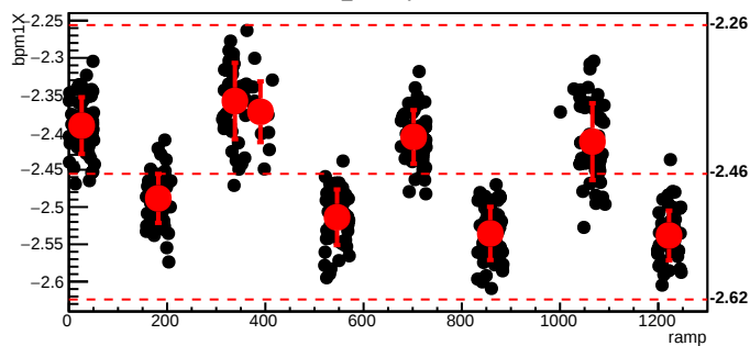
bmod_trim6,cyc=6764
