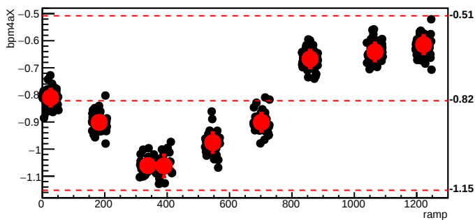
bmod_trim3,cyc=6764
