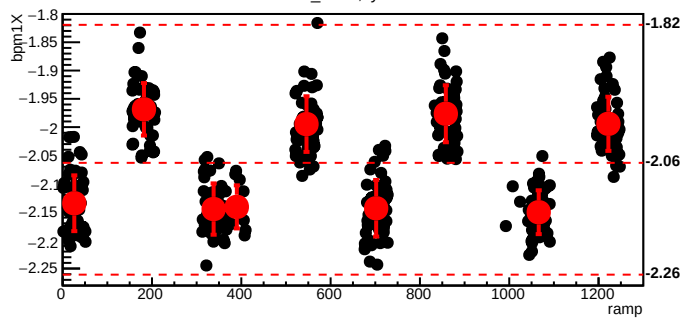
bmod_trim2,cyc=6785
