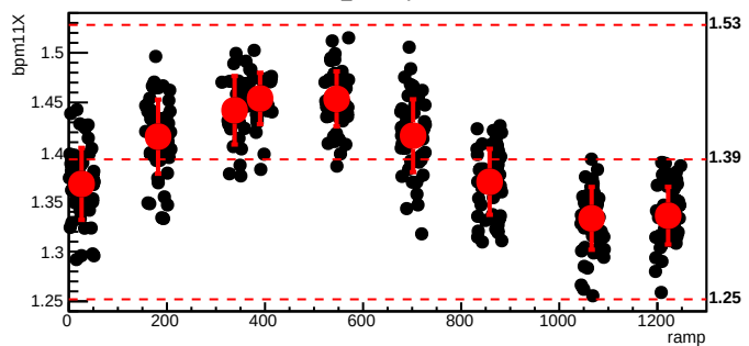
bmod_trim5,cyc=6785
