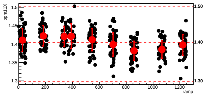
bmod_trim6,cyc=6785
