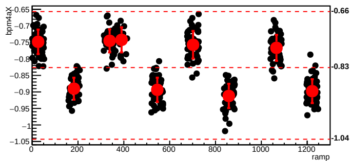
bmod_trim7,cyc=6785
