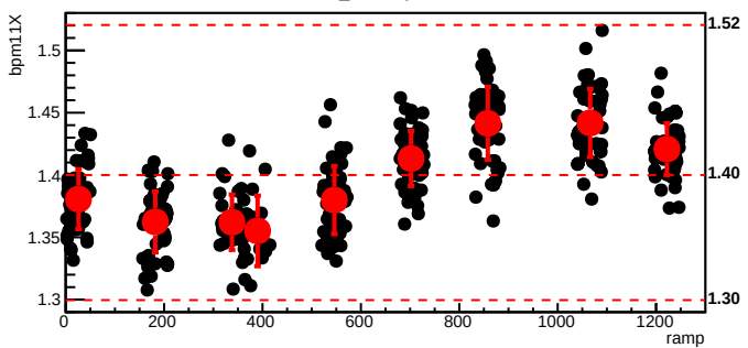
bmod_trim1,cyc=6785
