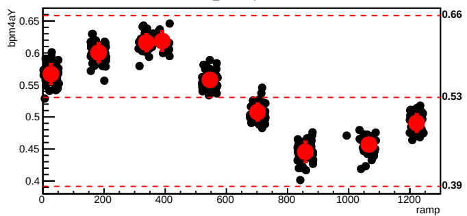
bmod_trim2,cyc=6785
