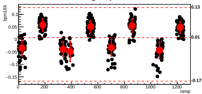
bmod_trim4,cyc=6785
