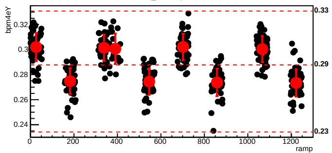
bmod_trim1,cyc=6785
