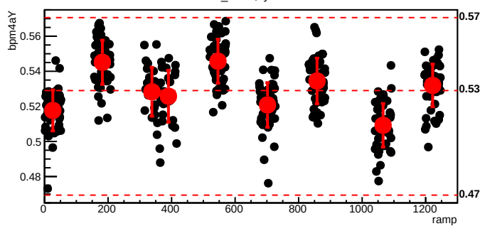
bmod_trim3,cyc=6785
