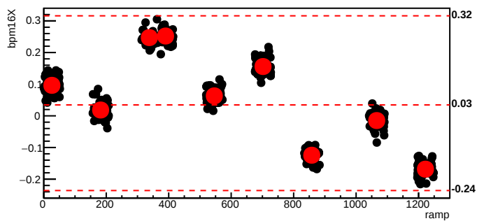
bmod_trim3,cyc=6788
