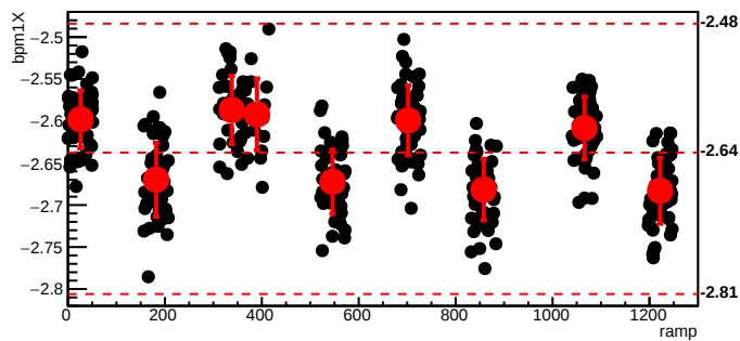
bmod_trim7,cyc=6788
