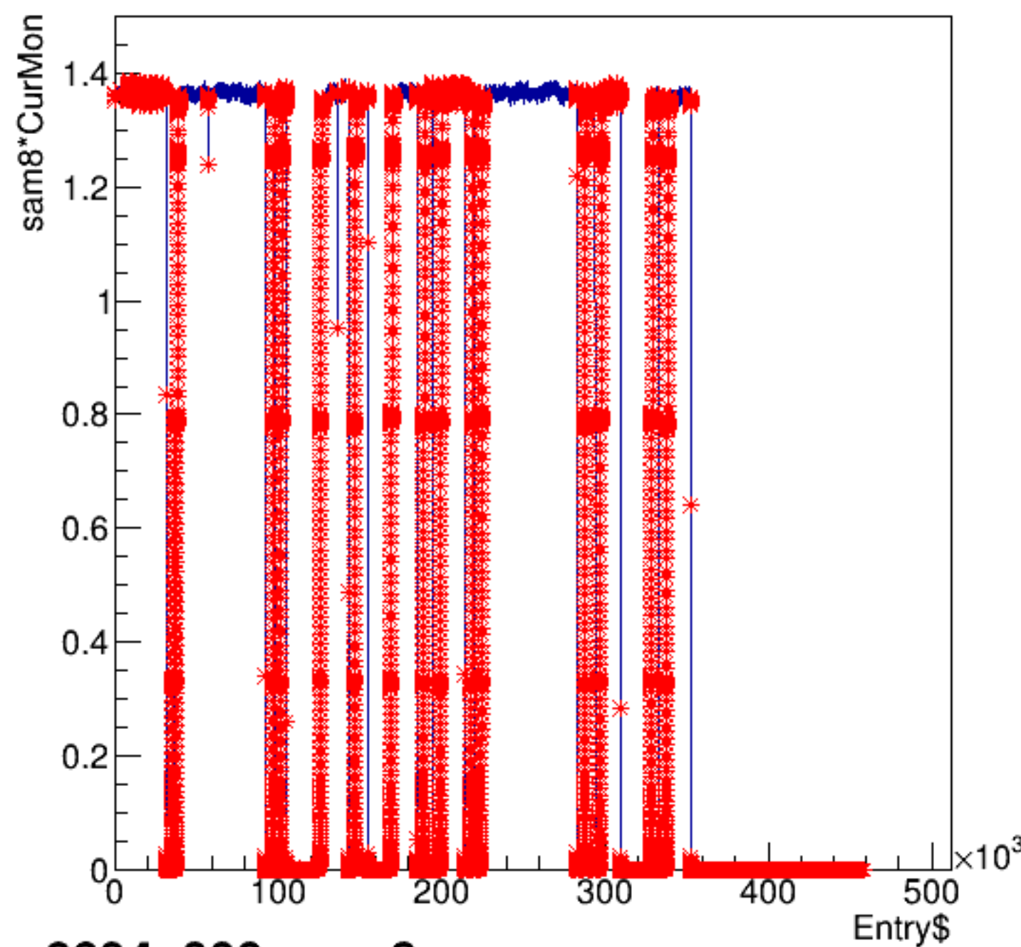
sam8*CurMon:Entry$
