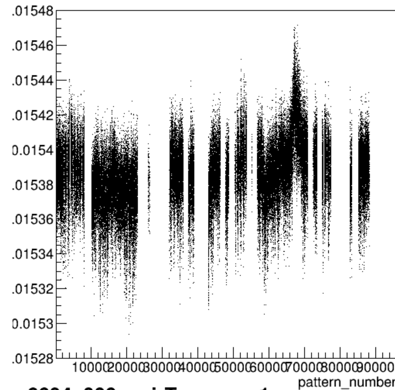
yield_sam1:pattern_number {ErrorFlag==0}
