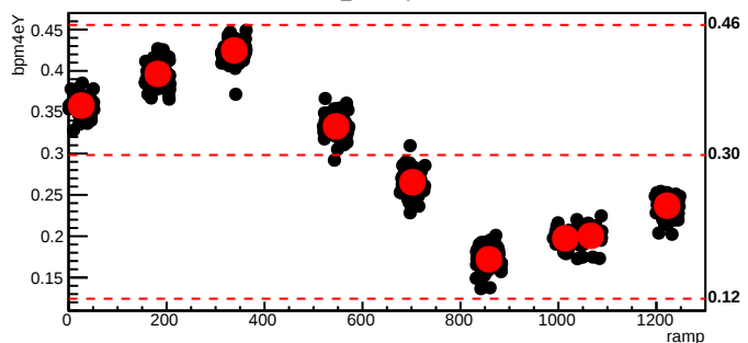
bmod_trim4,cyc=6850
