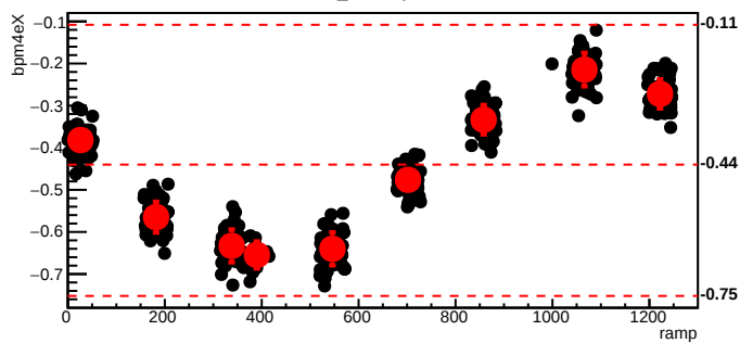
bmod_trim3,cyc=6883
