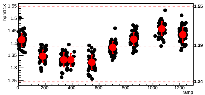
bmod_trim3,cyc=6883
