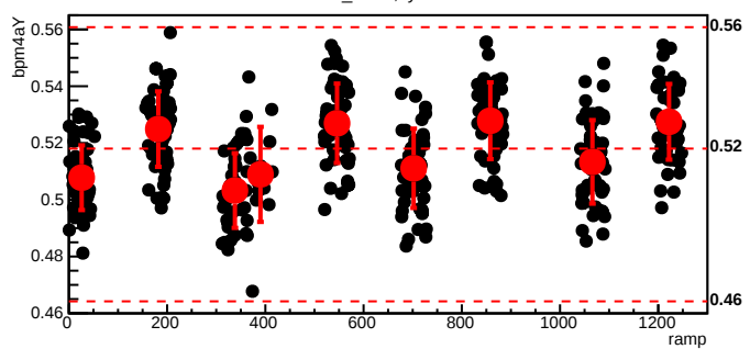
bmod_trim7,cyc=6883
