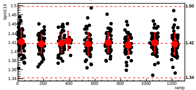
bmod_trim4,cyc=6883
