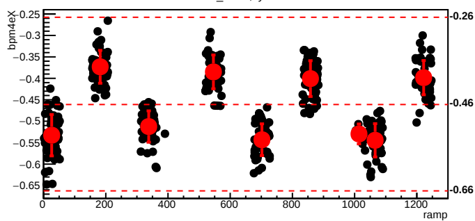
bmod_trim6,cyc=6883
