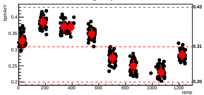
bmod_trim2,cyc=6883
