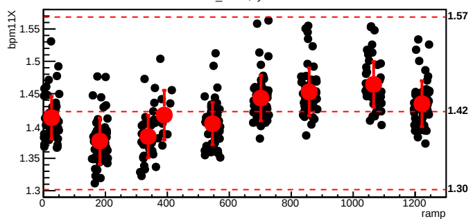
bmod_trim1,cyc=6883
