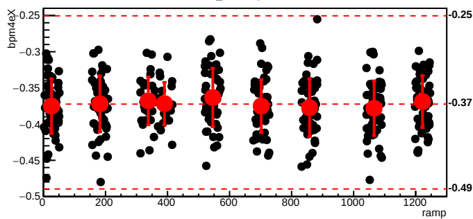
bmod_trim2,cyc=6927
