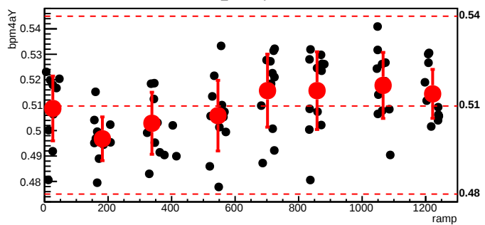
bmod_trim7,cyc=6927
