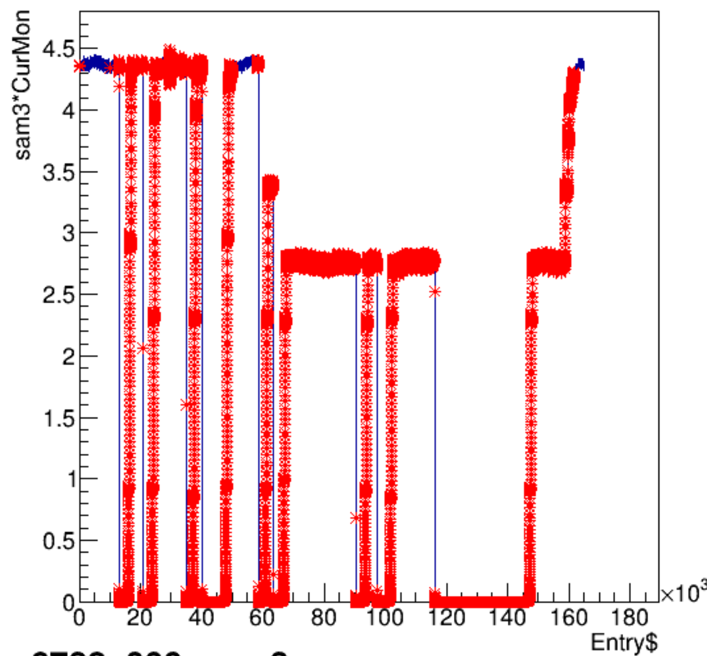
sam3*CurMon:Entry$
