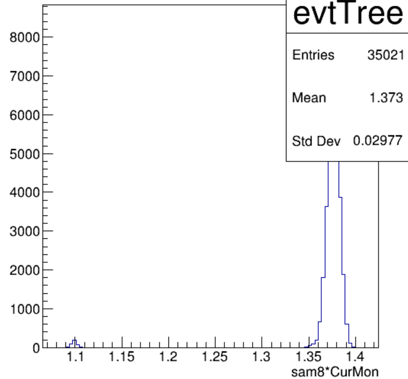
sam8*CurMon {ErrorFlag==0}
