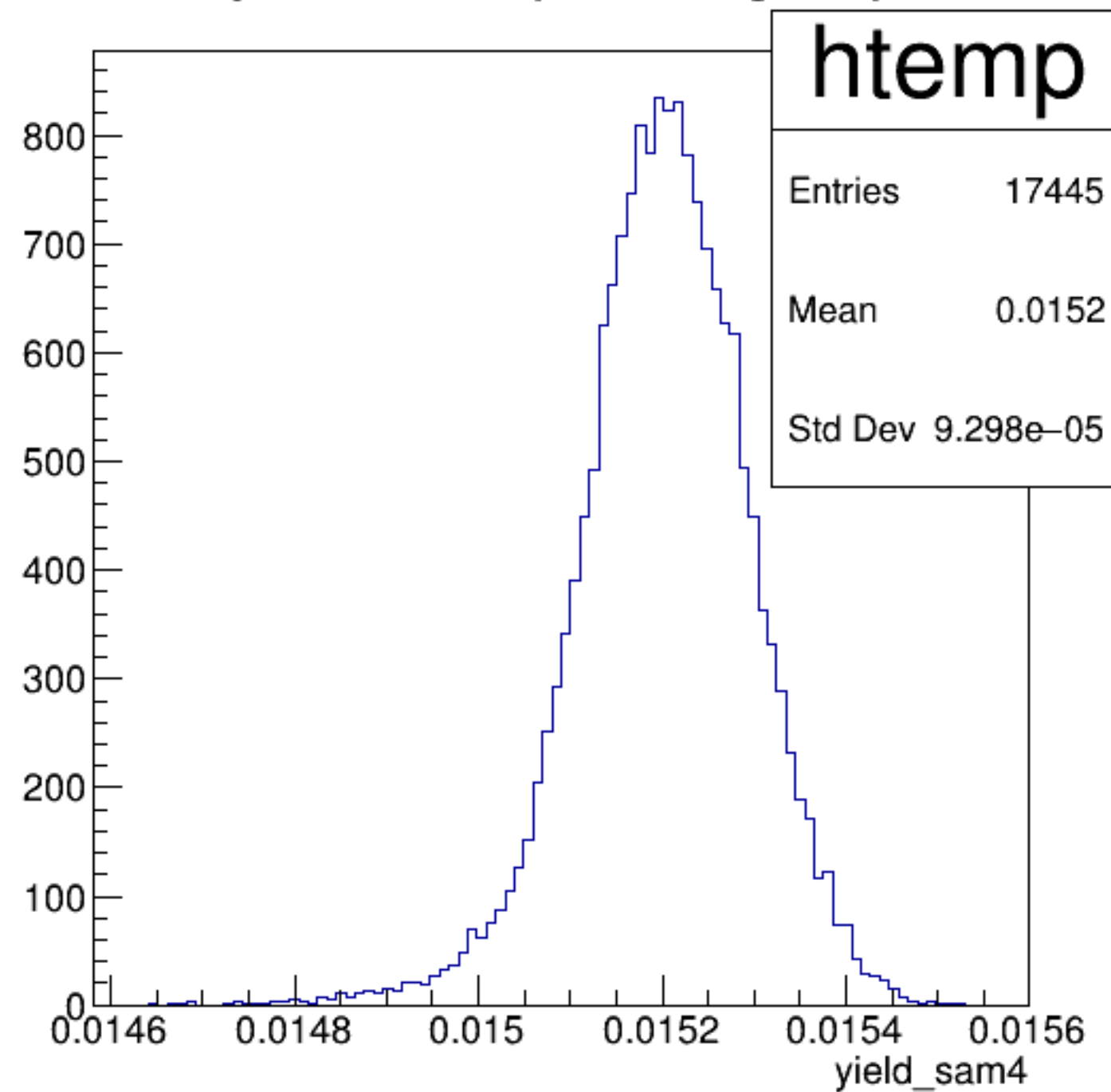
yield_sam4 {ErrorFlag==0}
