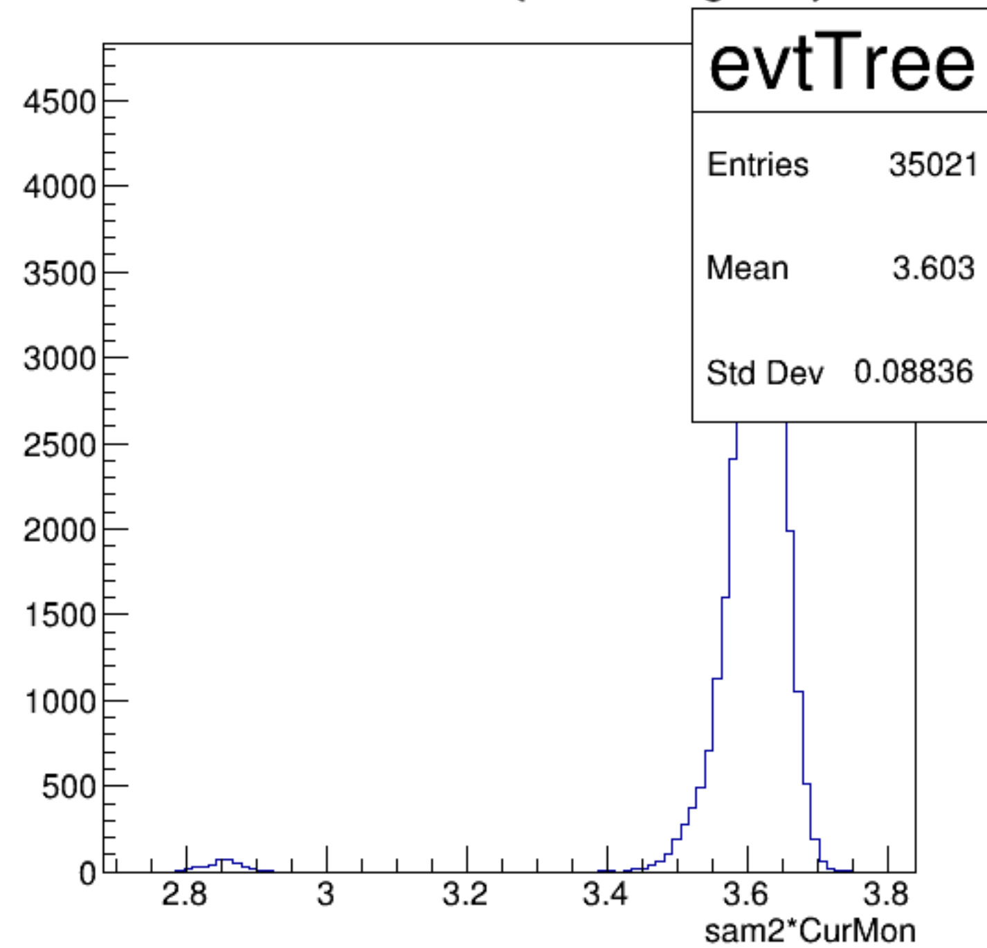
sam2*CurMon {ErrorFlag==0}
