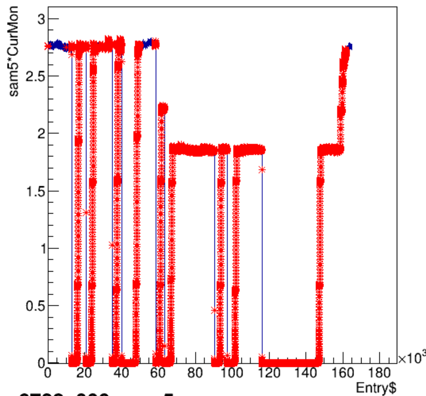
sam5*CurMon:Entry$
