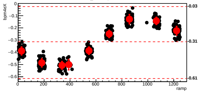
bmod_trim1,cyc=6963
