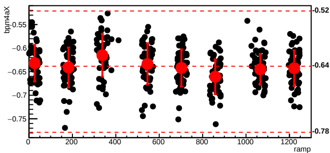
bmod_trim7,cyc=6963
