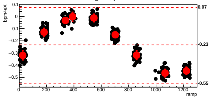
bmod_trim5,cyc=6963
