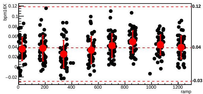
bmod_trim7,cyc=6963
