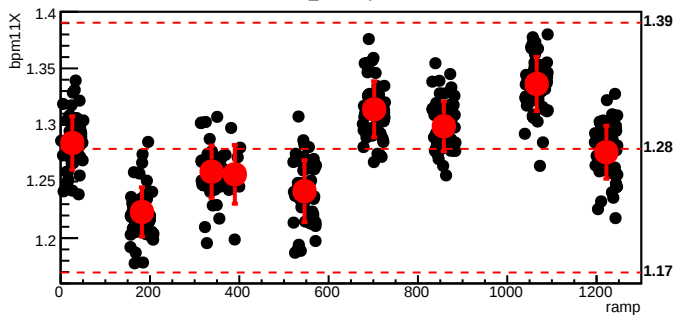
bmod_trim1,cyc=6963
