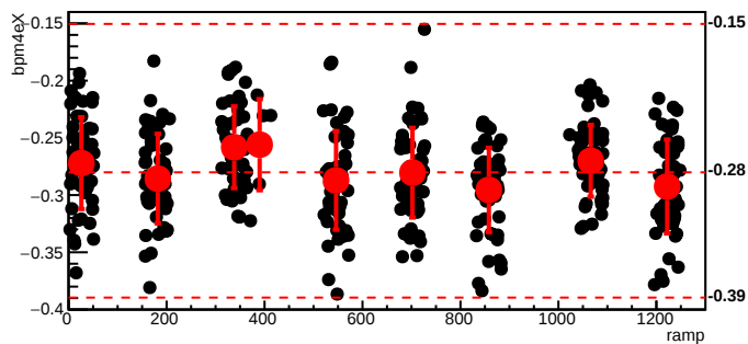
bmod_trim2,cyc=6963
