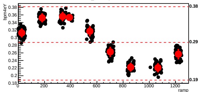
bmod_trim2,cyc=6963
