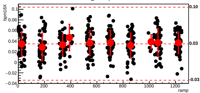
bmod_trim2,cyc=6994
