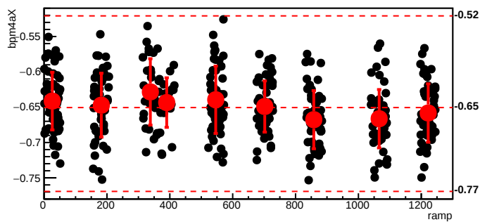
bmod_trim7,cyc=7048
