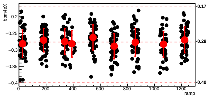
bmod_trim2,cyc=7048
