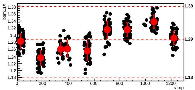
bmod_trim1,cyc=7048
