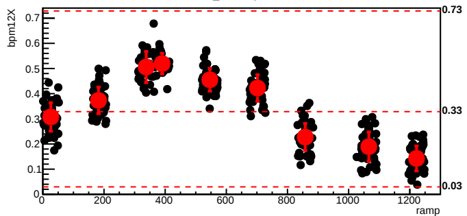
bmod_trim5,cyc=7048
