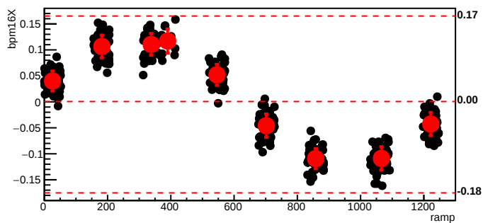
bmod_trim1,cyc=7048
