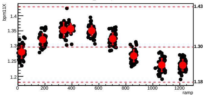
bmod_trim5,cyc=7048
