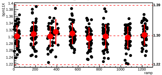
bmod_trim2,cyc=7048
