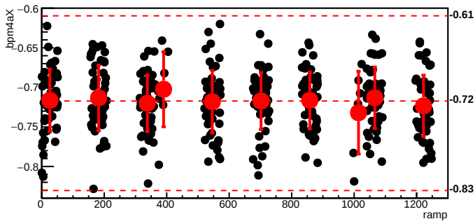
bmod_trim4,cyc=7054
