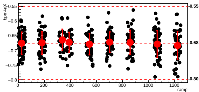
bmod_trim2,cyc=7054
