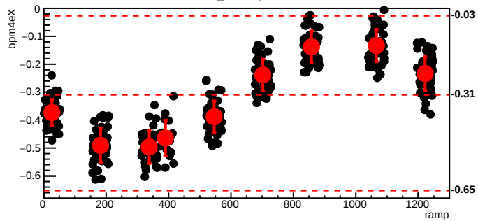
bmod_trim1,cyc=7054
