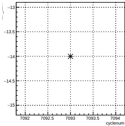
4eY_coil7:cyclenum {run == 6818}
