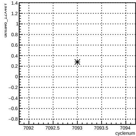
delta46_12X4eY:cyclenum {run == 6818}
