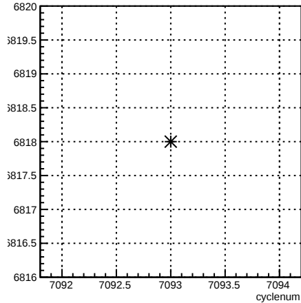
run:cyclenum {run == 6818}
