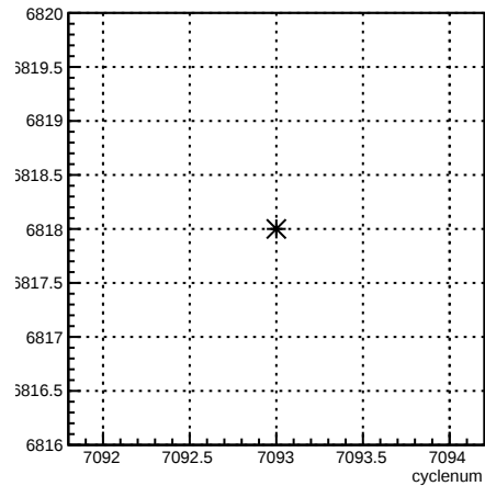
run:cyclenum {run == 6818}
