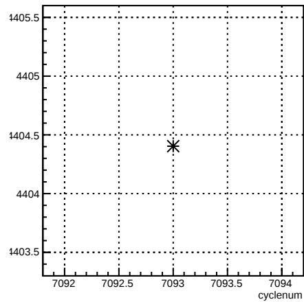
run:cyclenum {run == 6818}
