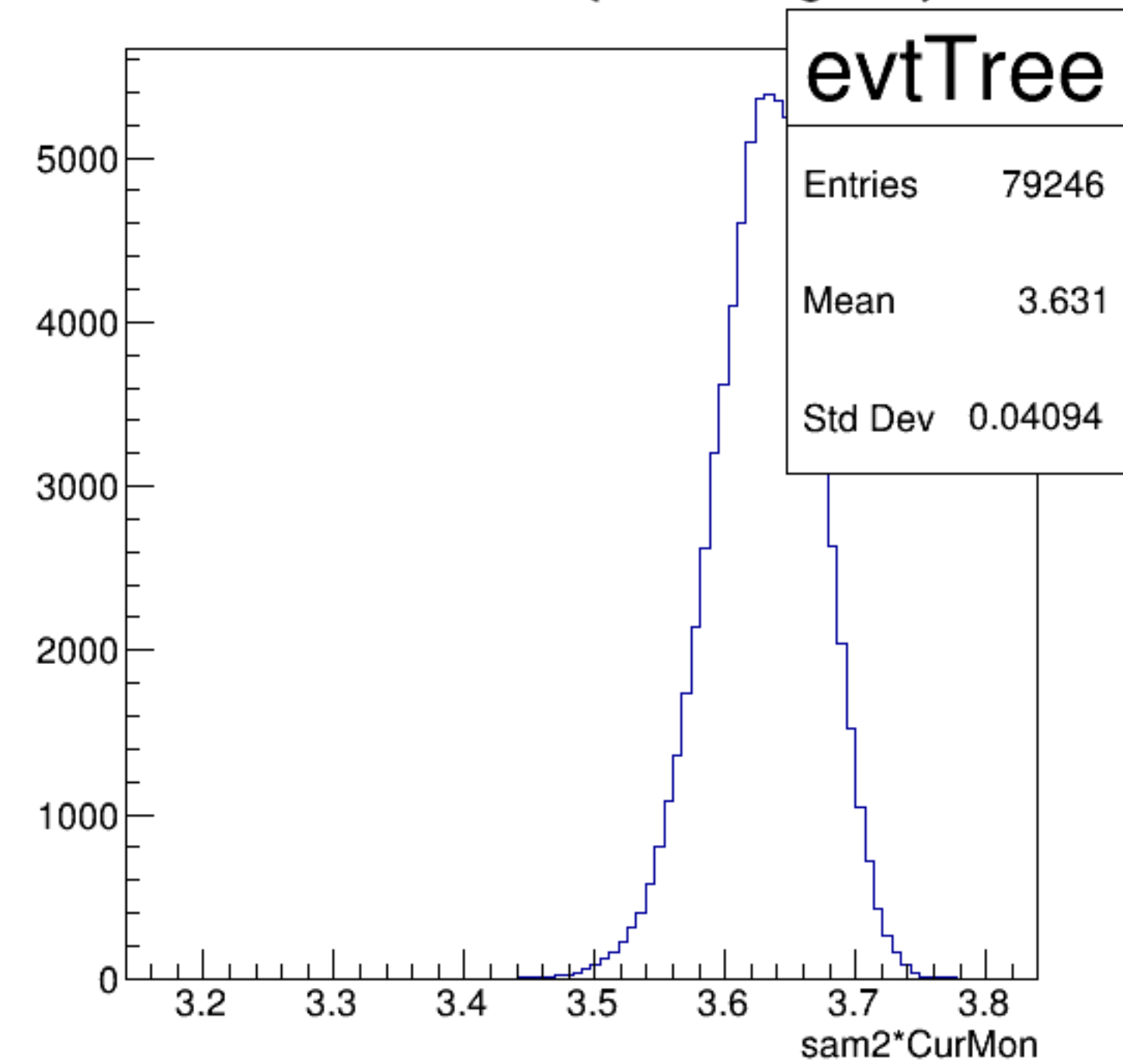
sam2*CurMon {ErrorFlag==0}
