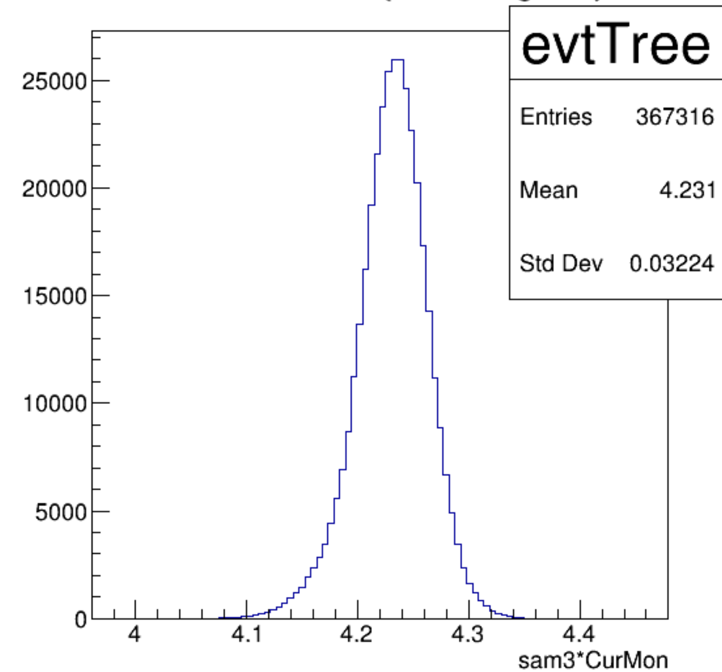
sam3*CurMon {ErrorFlag==0}
