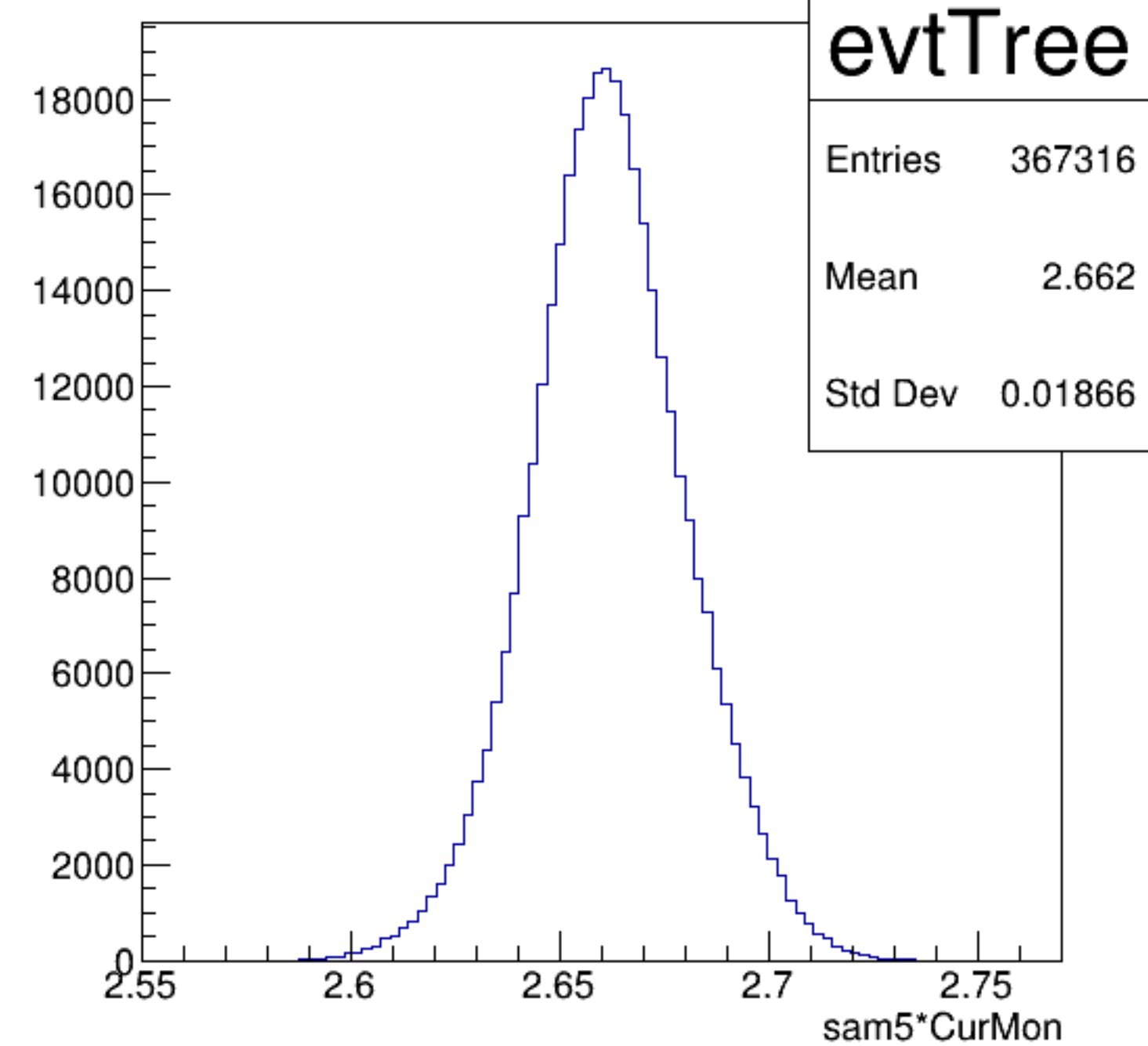
sam5*CurMon {ErrorFlag==0}
