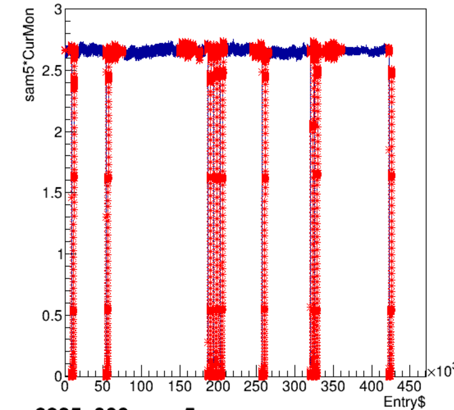
sam5*CurMon:Entry$
