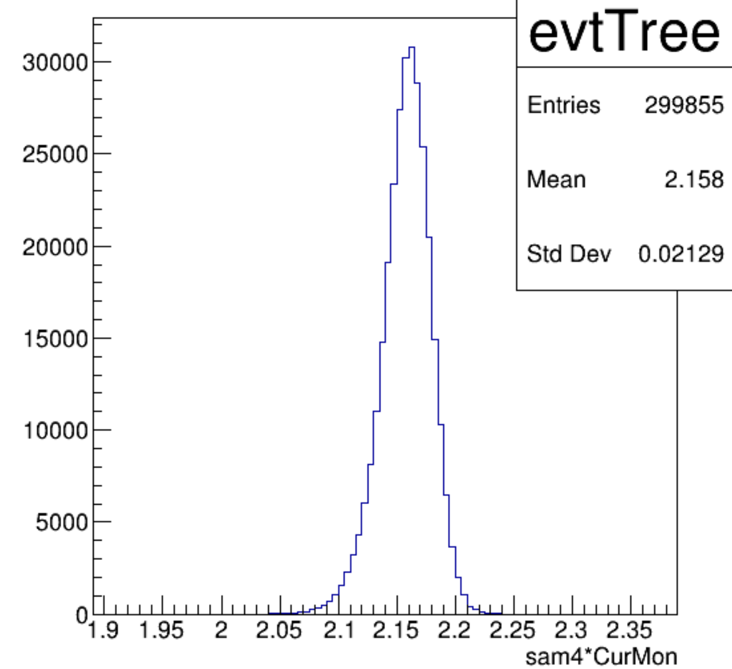
sam4*CurMon {ErrorFlag==0}
