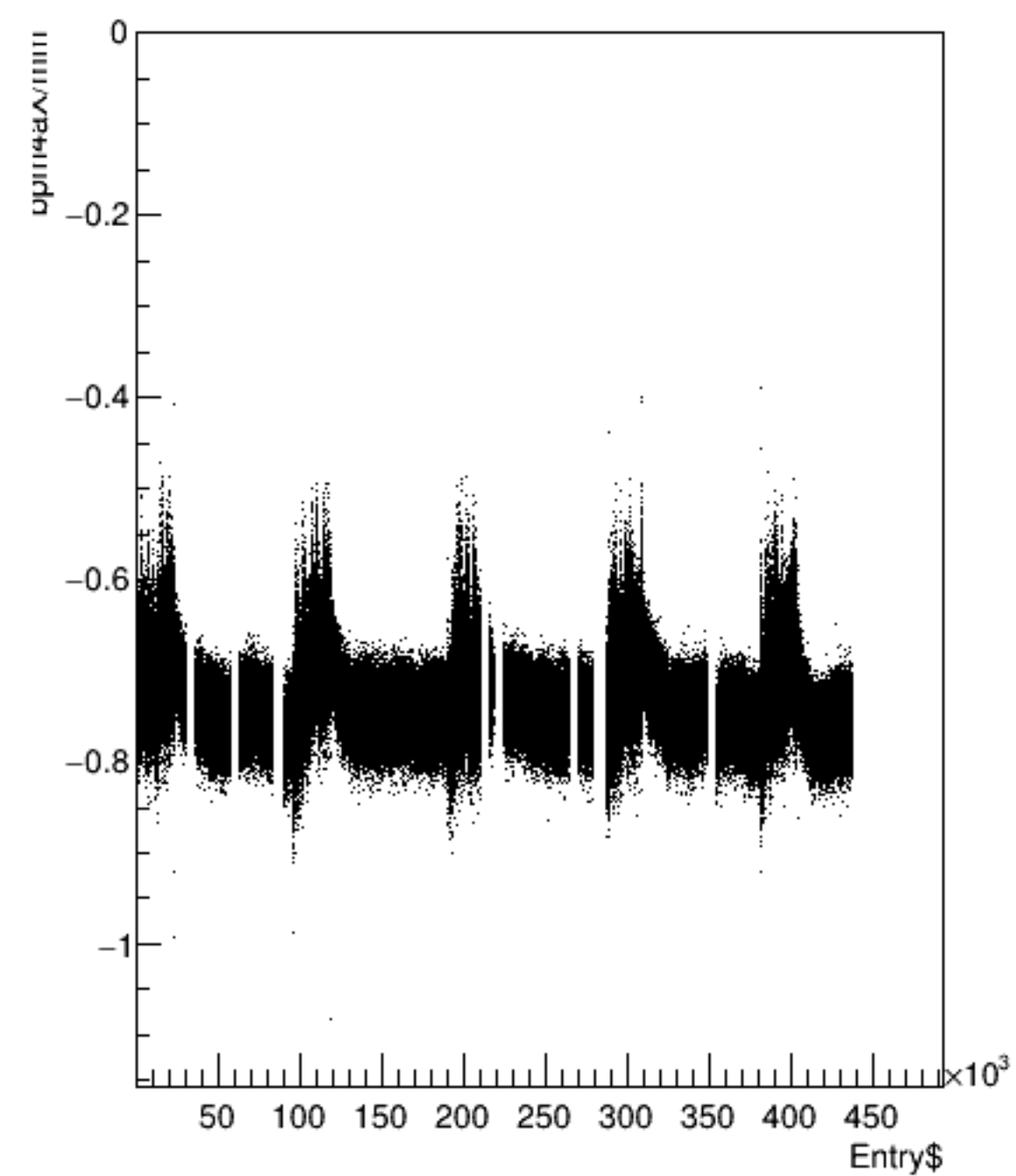
bpm4aX/mm:Entry$ {ErrorFlag==0}
