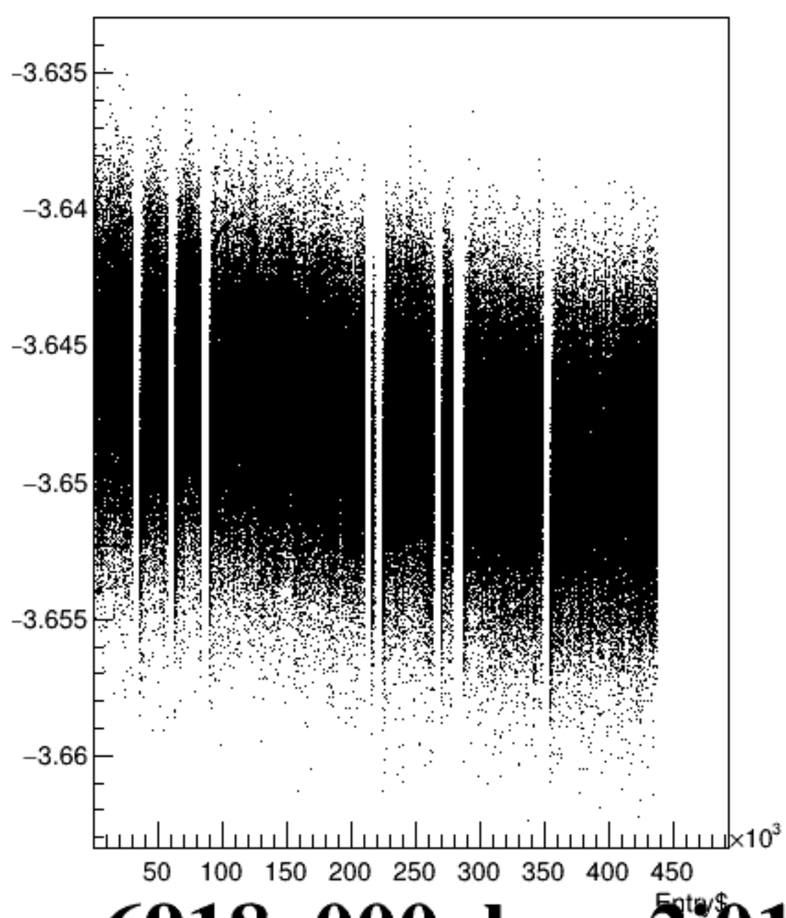
bpm2i01Y/mm:Entry$ {ErrorFlag==0}
