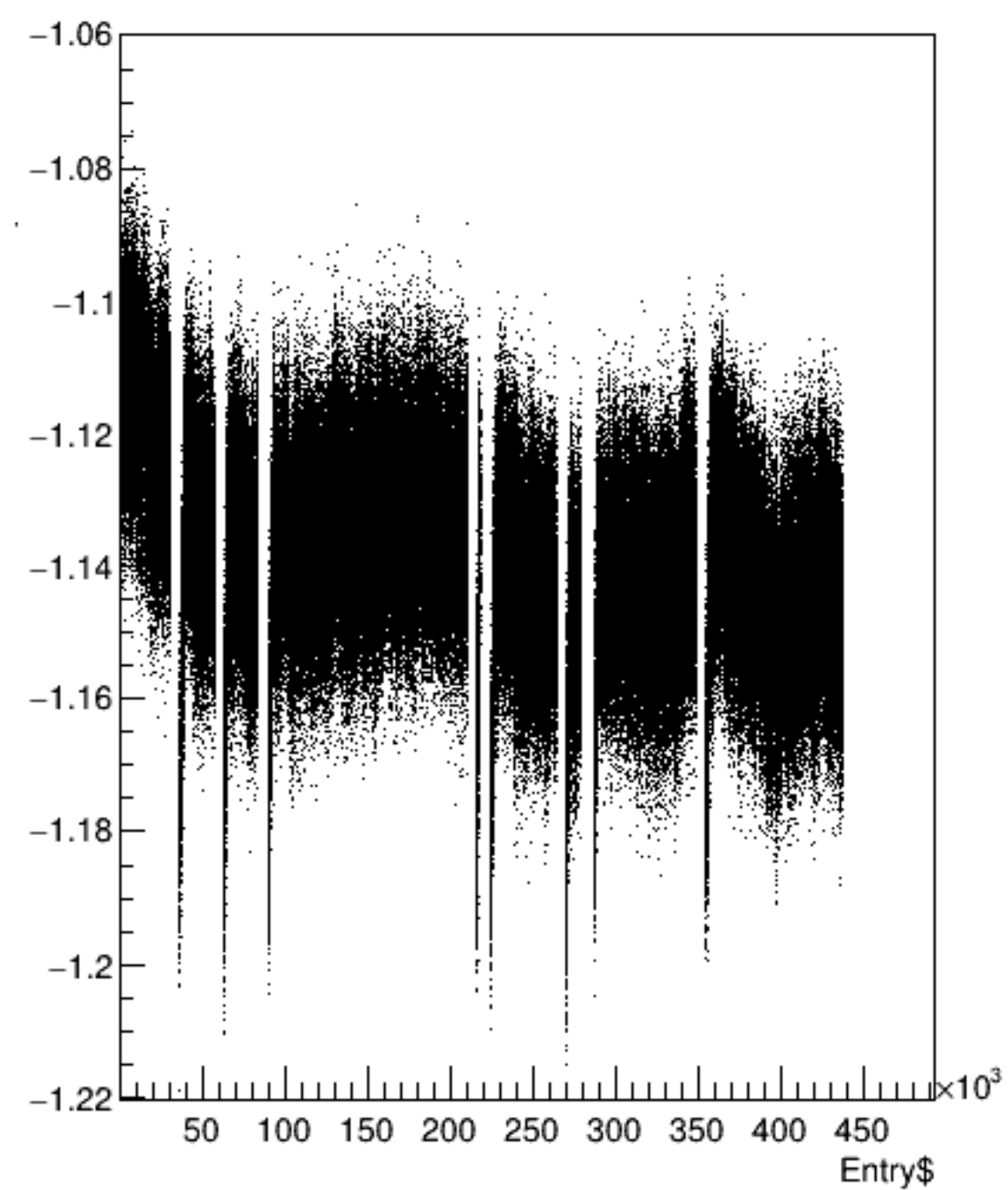
bpm0I01X/mm:Entry$ {ErrorFlag==0}
