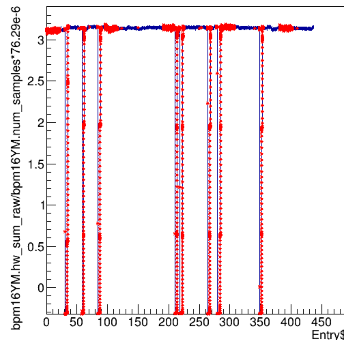
bpm16YM.hw_sum_raw/bpm16YM.num_samples*76.29e-6:Entry$
