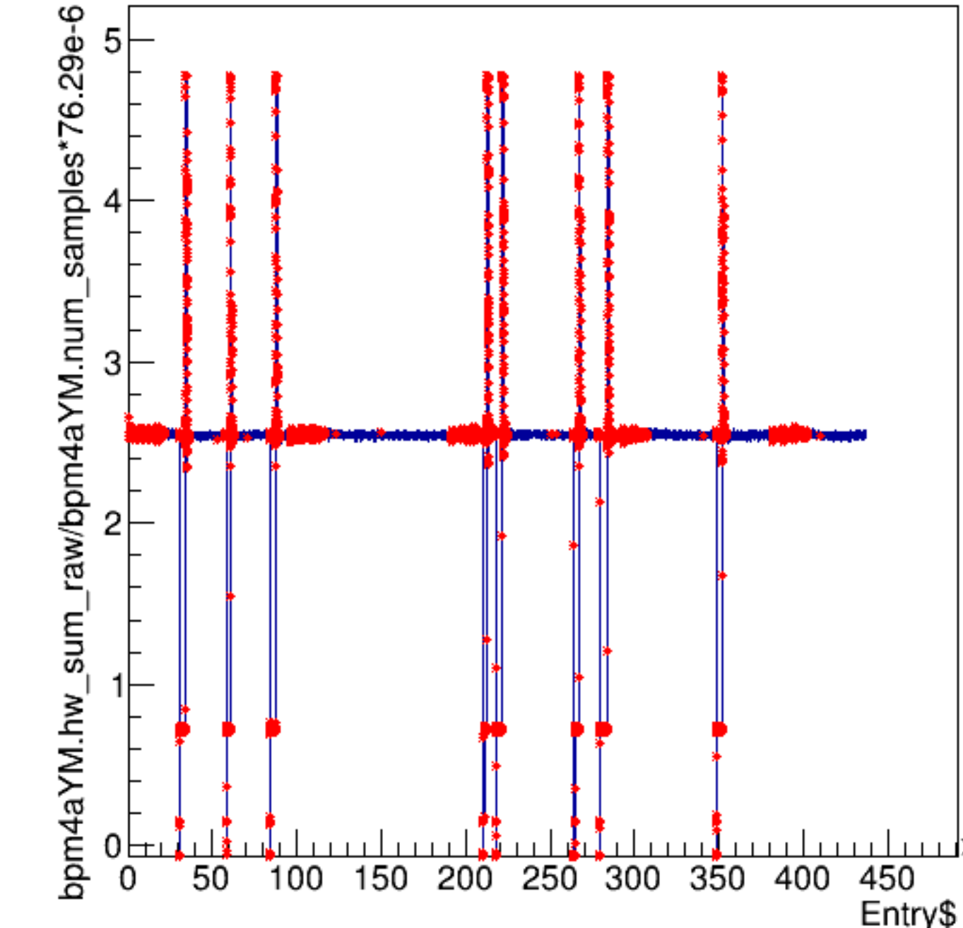
bpm4aYM.hw_sum_raw/bpm4aYM.num_samples*76.29e-6:Entry$
