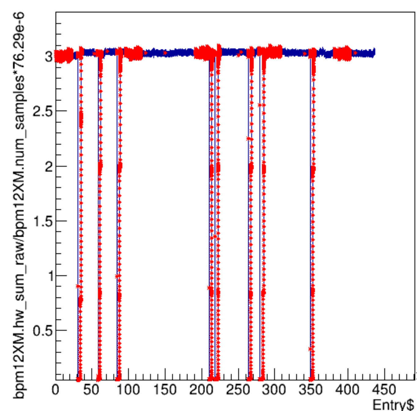
bpm12XM.hw_sum_raw/bpm12XM.num_samples*76.29e-6:Entry$
