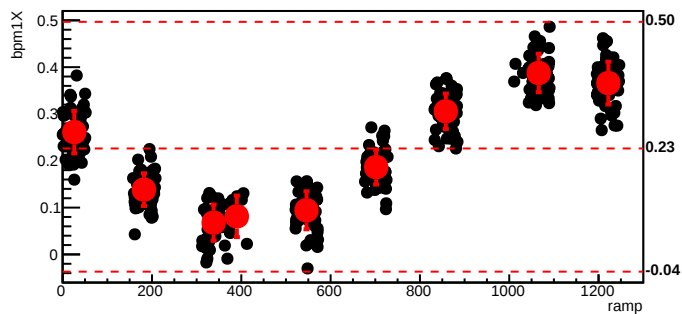
bmod_trim3,cyc=7317
