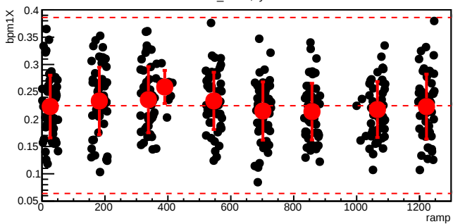
bmod_trim6,cyc=7317
