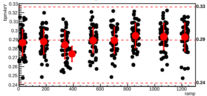
bmod_trim7,cyc=7317
