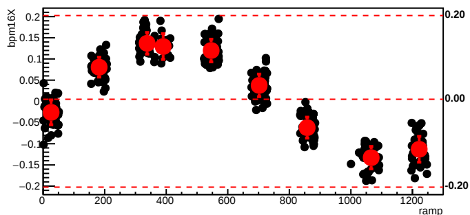
bmod_trim3,cyc=7317
