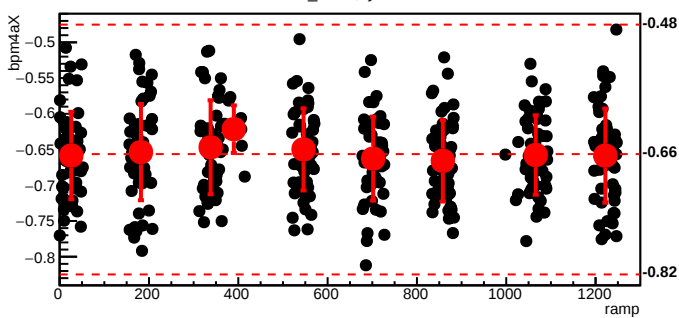
bmod_trim6,cyc=7317
