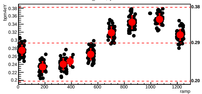
bmod_trim6,cyc=7317
