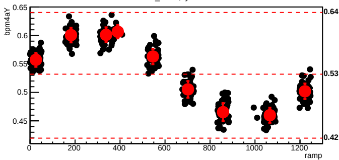
bmod_trim6,cyc=7317
