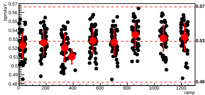
bmod_trim7,cyc=7317
