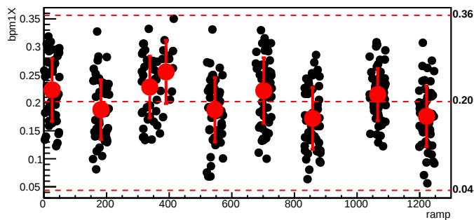
bmod_trim6,cyc=7340
