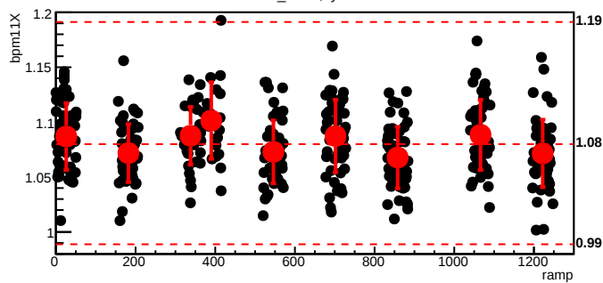
bmod_trim2,cyc=7340
