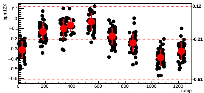
bmod_trim5,cyc=7340
