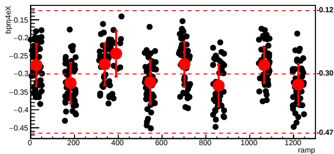
bmod_trim6,cyc=7340
