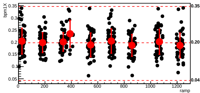
bmod_trim2,cyc=7437
