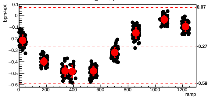
bmod_trim3,cyc=7437
