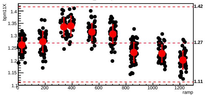
bmod_trim5,cyc=7437
