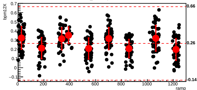
bmod_trim2,cyc=7437
