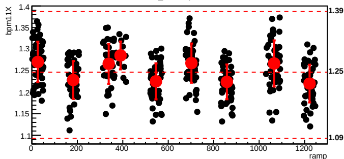
bmod_trim2,cyc=7437
