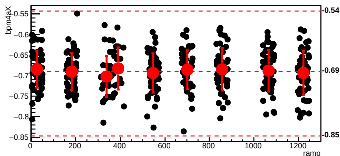
bmod_trim4,cyc=7437
