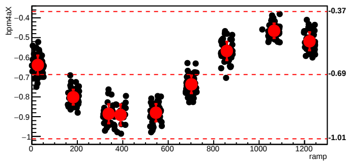
bmod_trim3,cyc=7437
