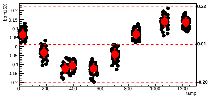
bmod_trim5,cyc=7437
