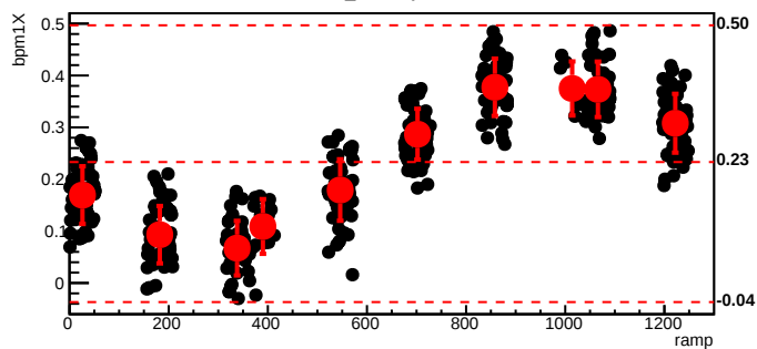
bmod_trim1,cyc=7437
