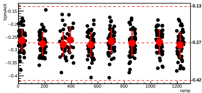
bmod_trim4,cyc=7437
