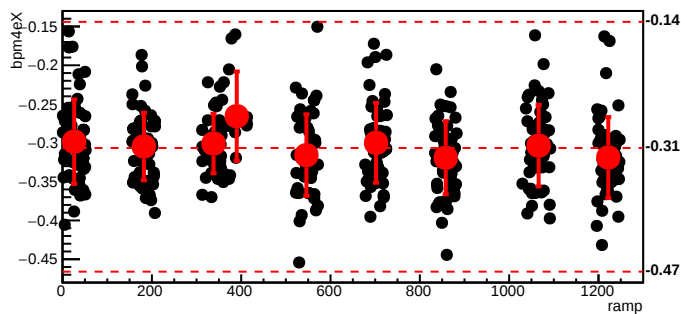
bmod_trim2,cyc=7437
